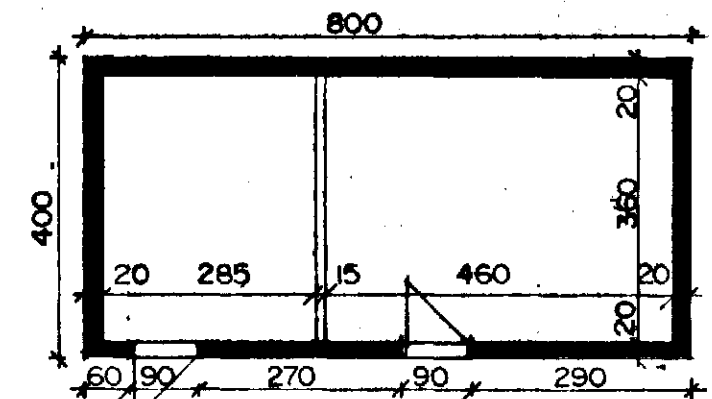
GRUNNMYND M. 1:100
