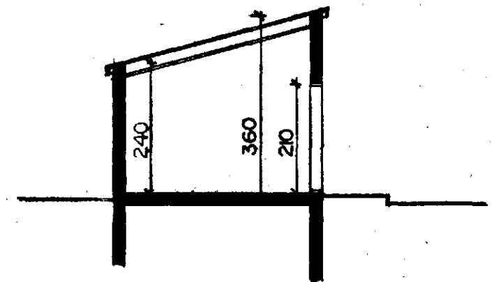
SNÍÐ M. 1:100
