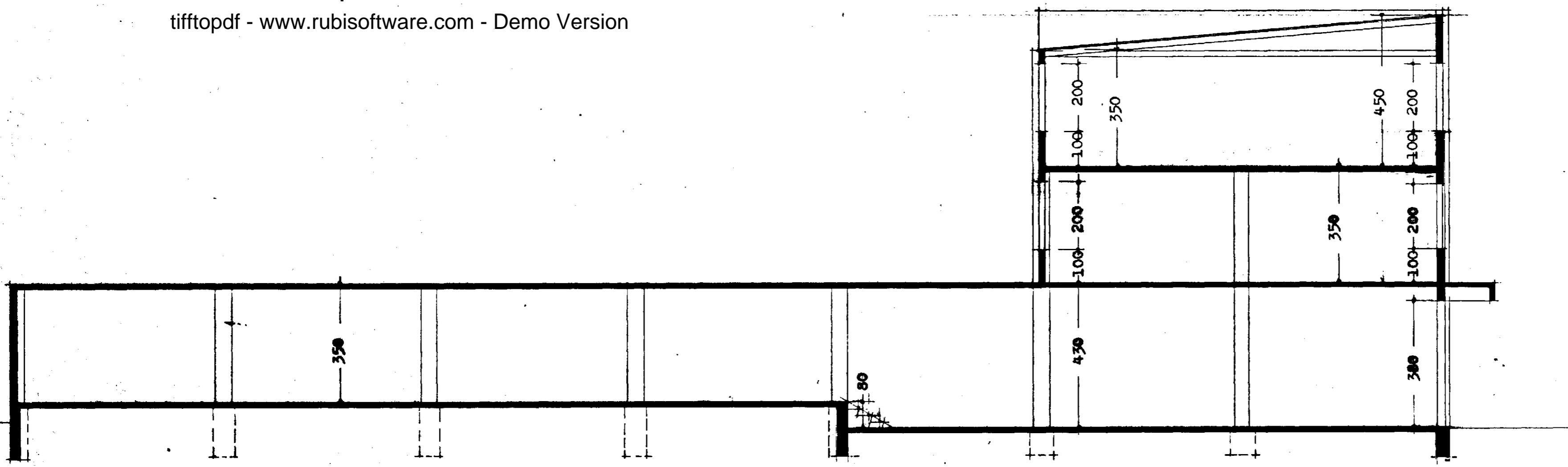
skurður A-A
