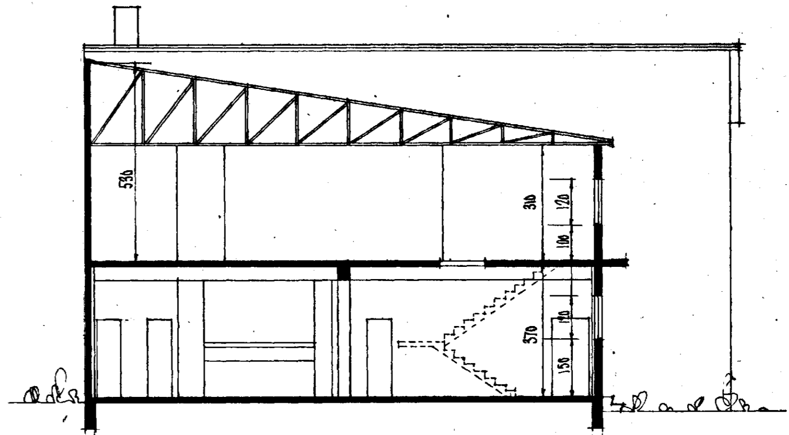
SNID: A-A
