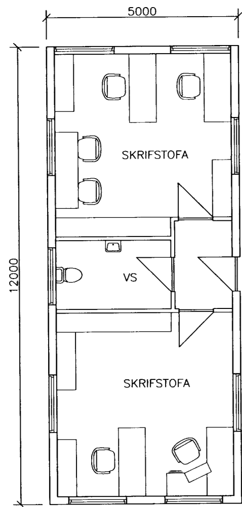
NÝ VERKSTJÓRAADASTADA GRUNNMYND 1:100
