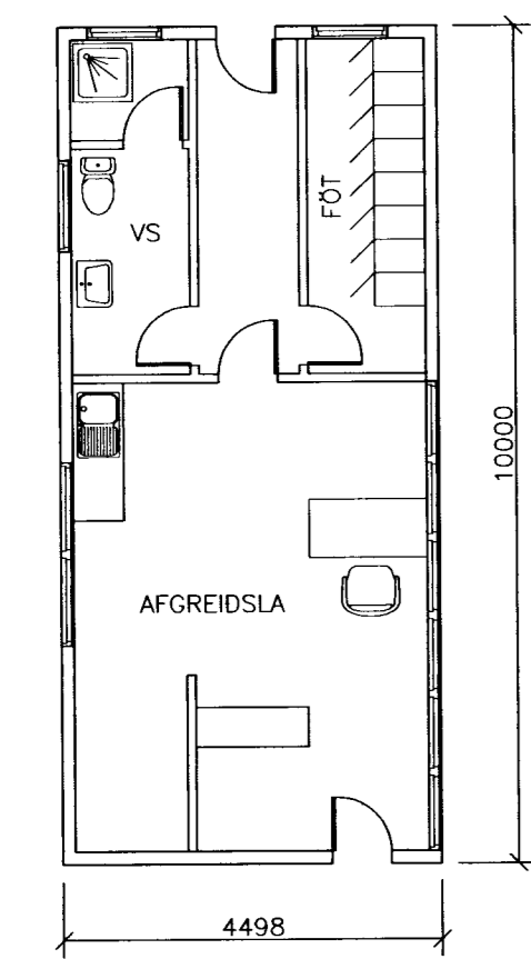
SKRIFSTOFA GRUNNMYND 1:100
