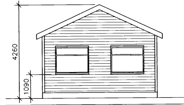
SUDURHLID
