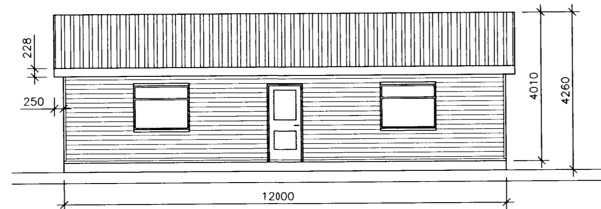
AUSTURHLID
