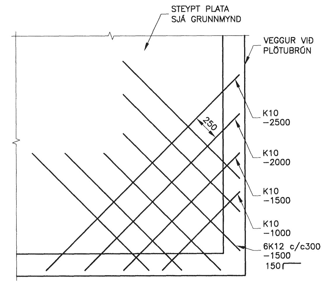
D52 JÁRNBENDING Í PLÖTUHORN MKV. 0
