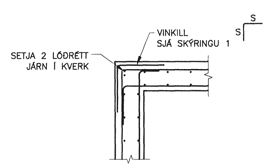
D02 DÆMIGERD JÁRNBENDING Í SAMSEYKTUM VEGGJA OG PLATNA – LÁRÉTT SNIÐ MKV. 0
