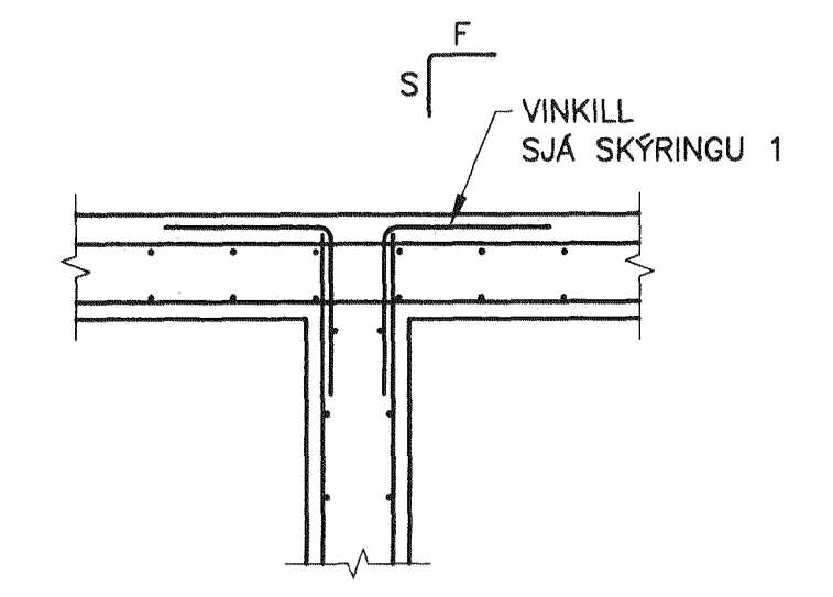
D02 DÆMIGERD JÁRNBENDING Í SAMSEYKTUM VEGGJA OG PLATNA – LÁRÉTT SNIÐ MKV. 0
