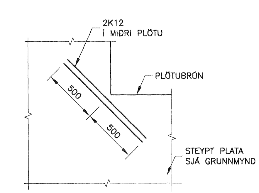
D51 JÁRNBENDING Í PLÖTUHORN MKV. 0
