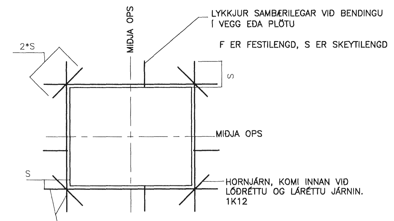
D53 JÁRNBENDING UMVERFIS ÖP MKV. 0
