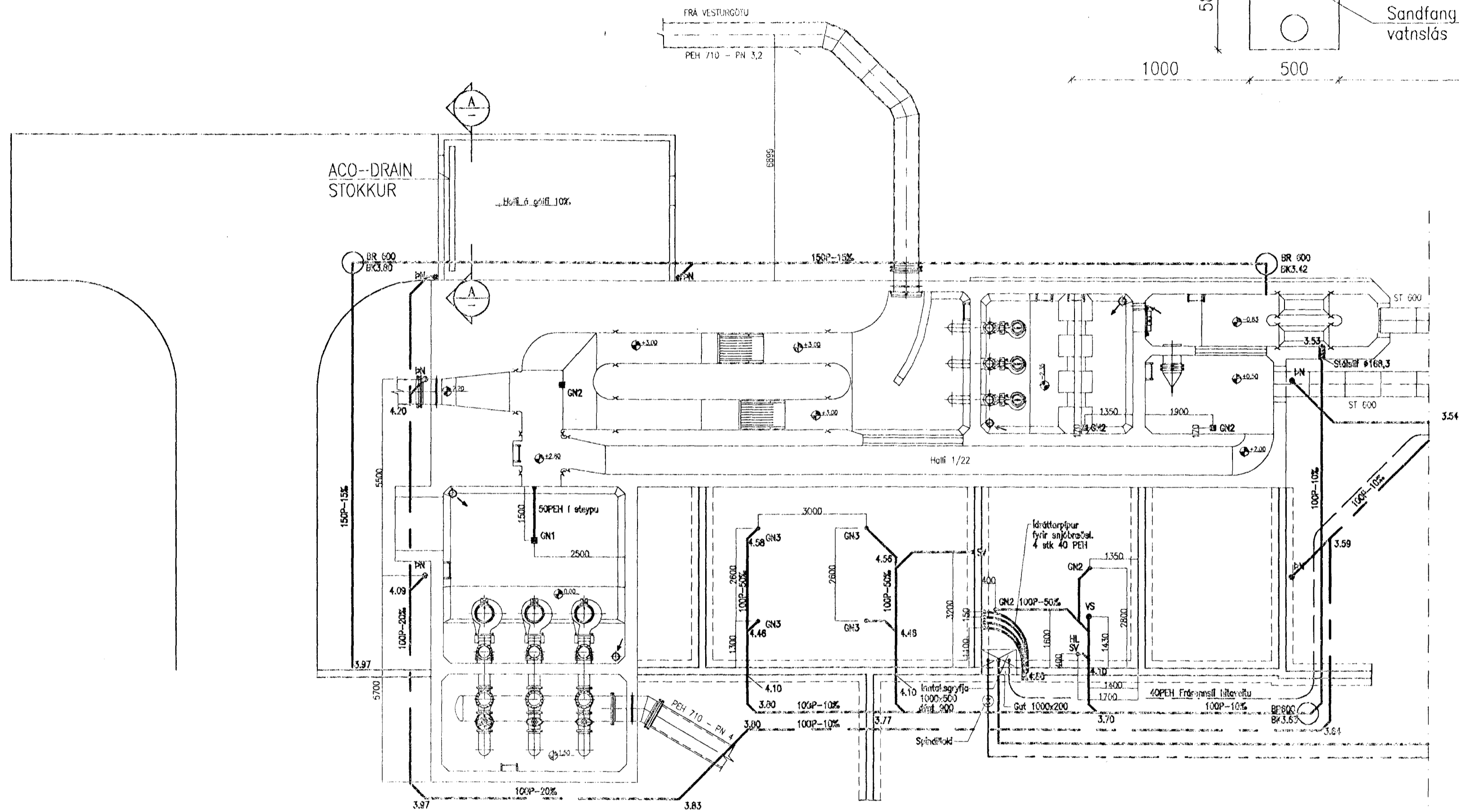
GRUNNMYND NEDRI HÆÐAR 1:100
