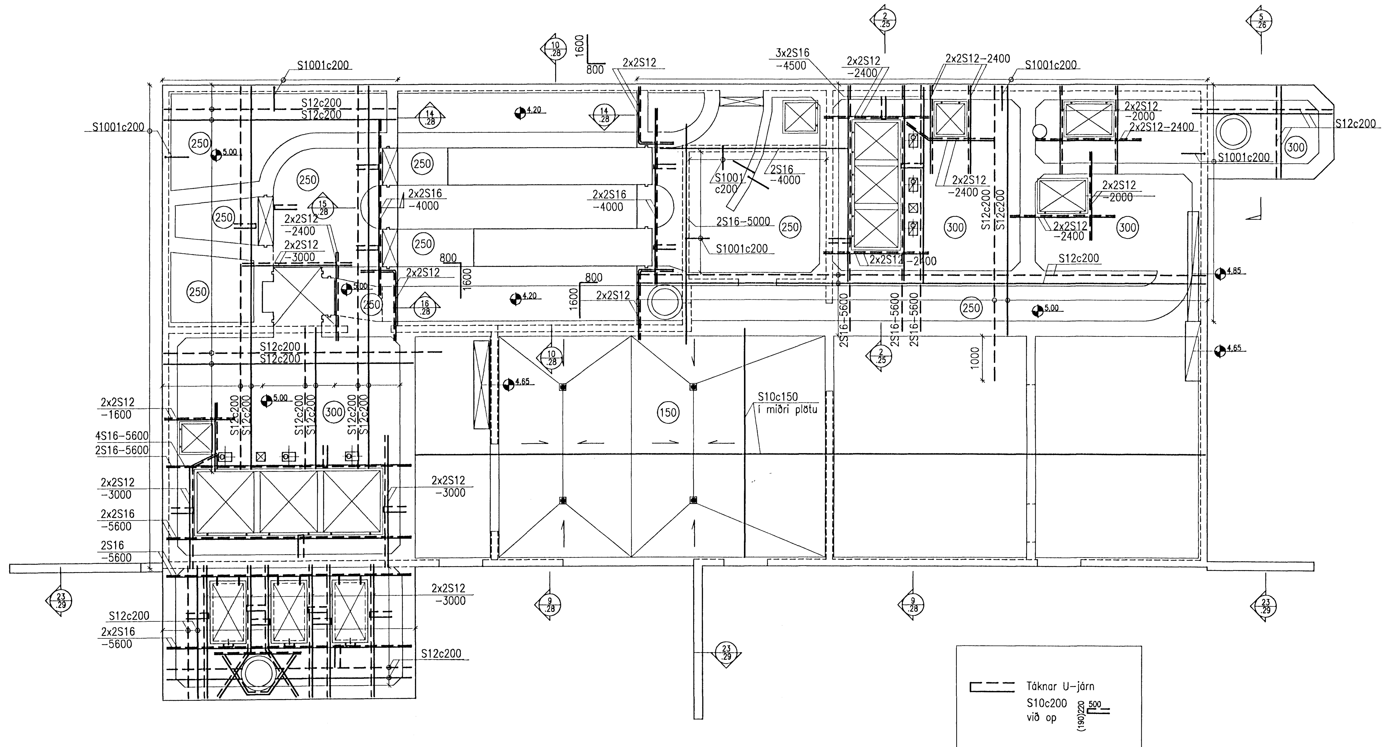
GRUNNMYND HÆÐ +5.0
