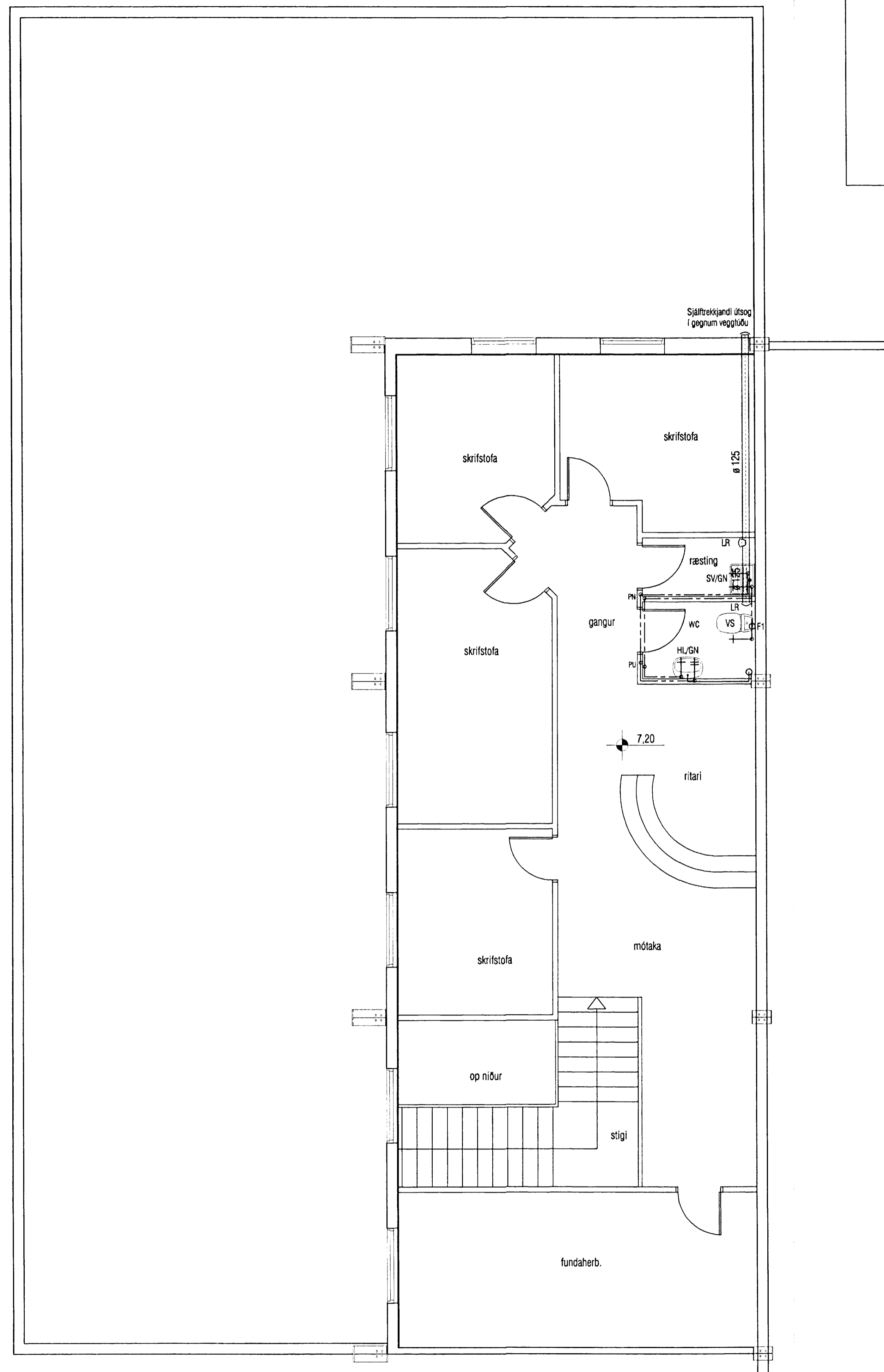
GRUNNMYND 2. HÆÐAR mkv. 1:50
