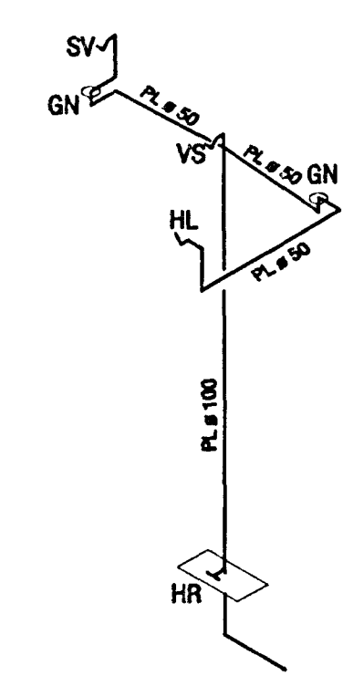
RÚMMYND FALLSTAMMA F1 mkv. 1:50
