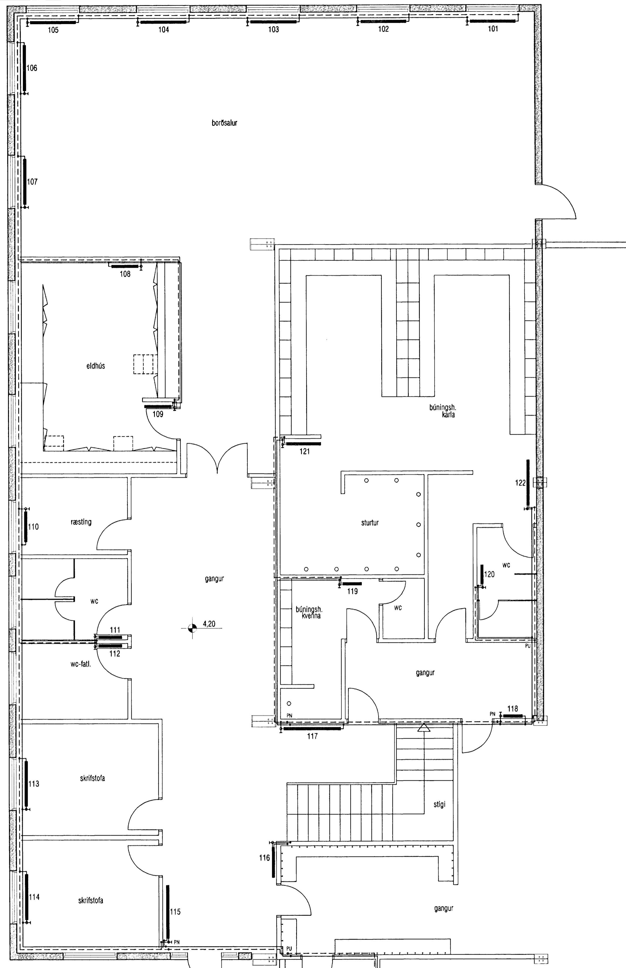
GRUNNMYND 1. HÆÐAR mkv. 1:50
