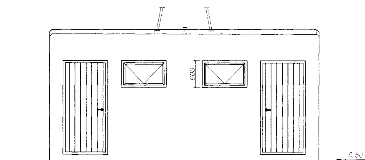
Norðurhlíð Mælikvarði 1:50
