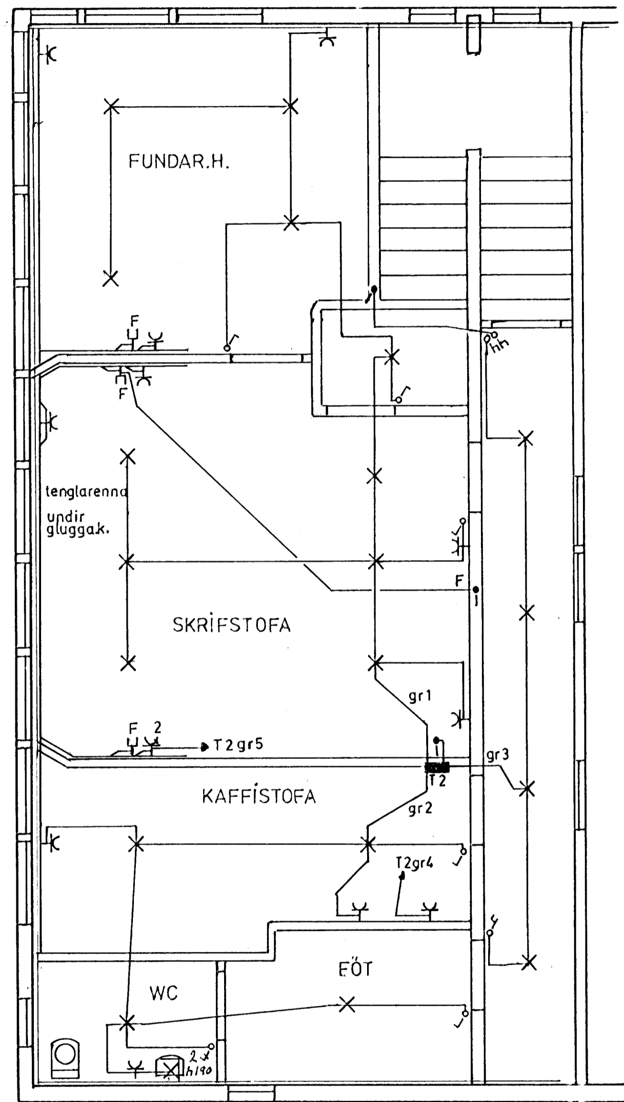
EFRI HÆÐ
