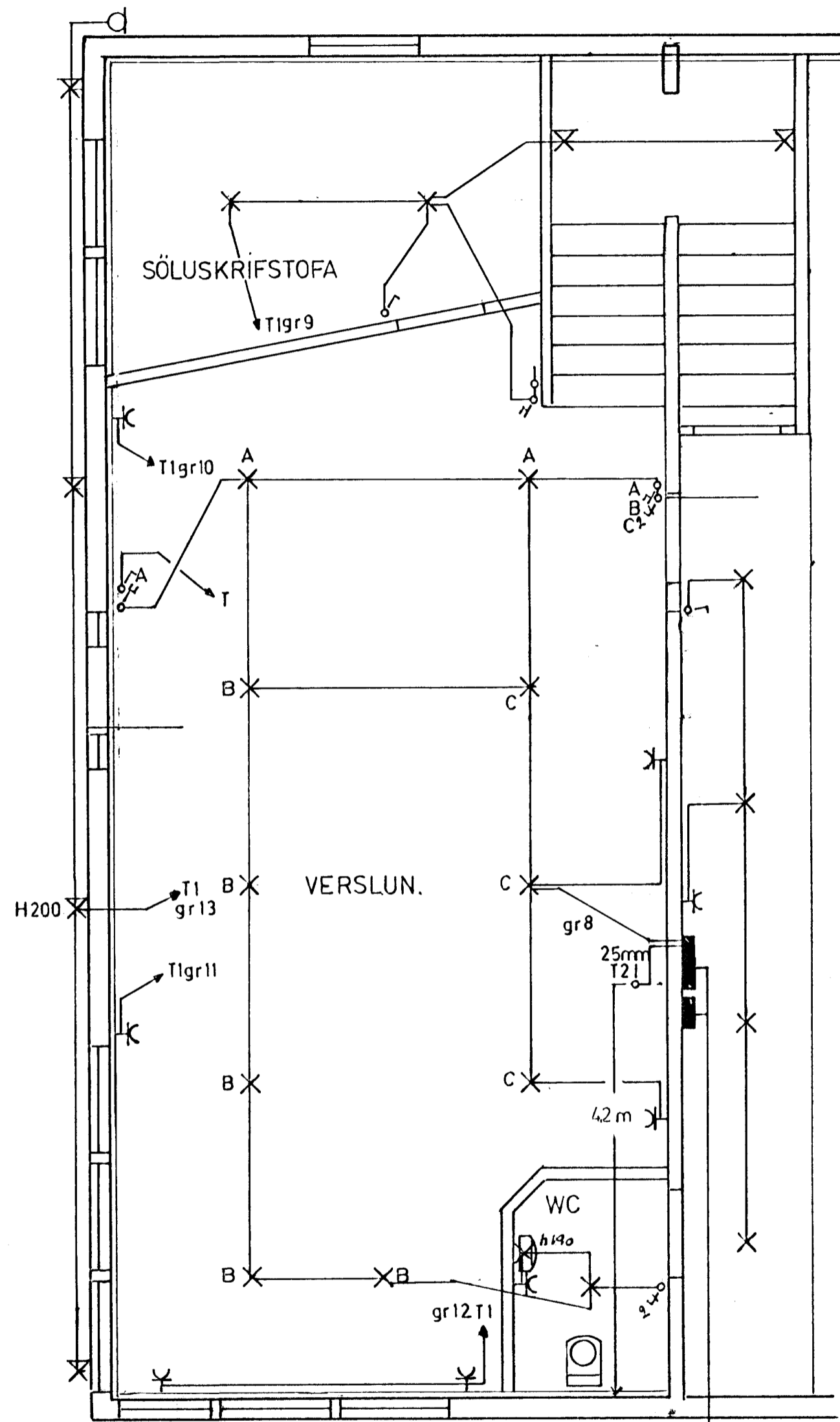
NEÐRI HÆÐ
