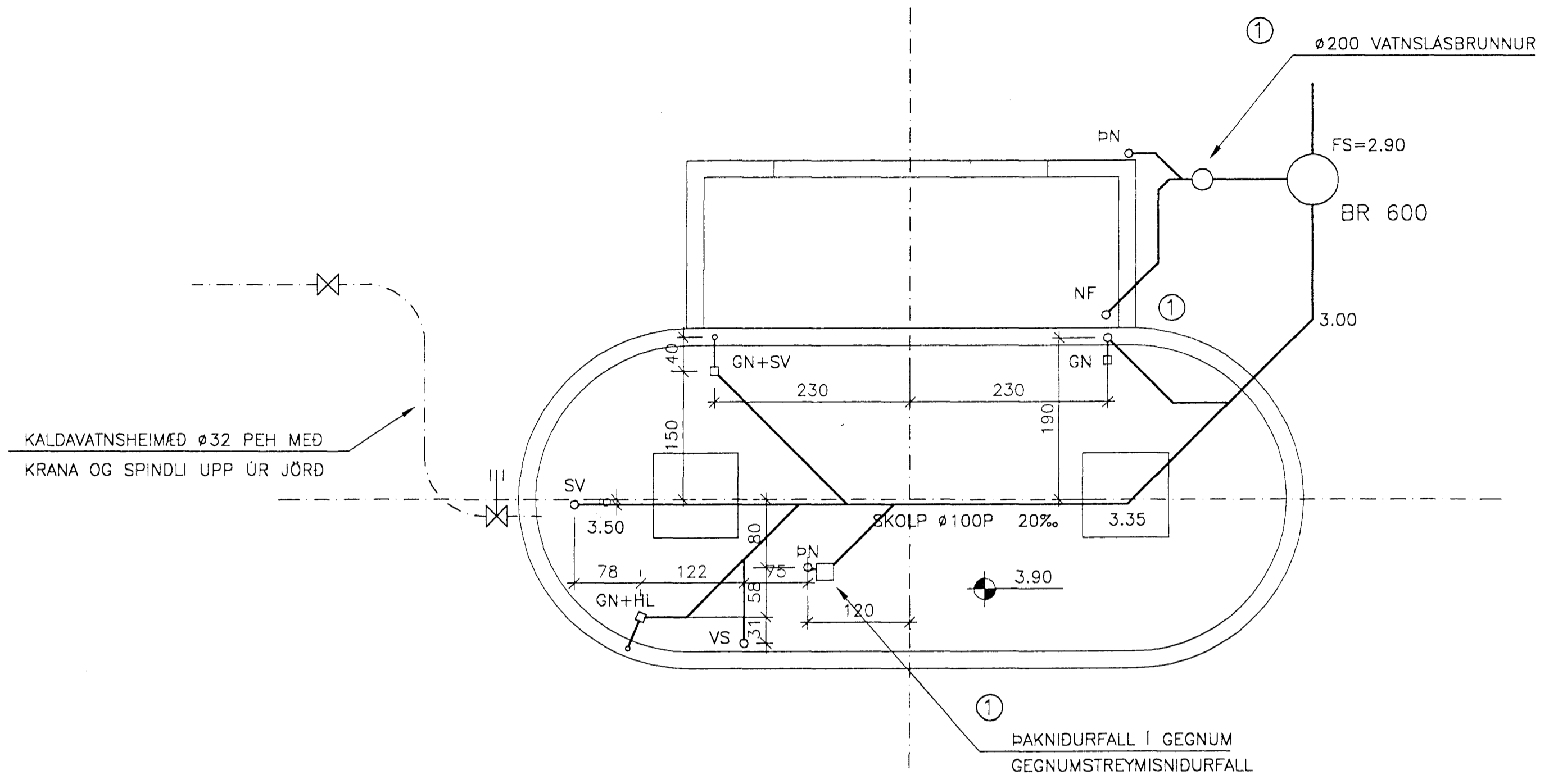
GRUNNMYND 1:50
