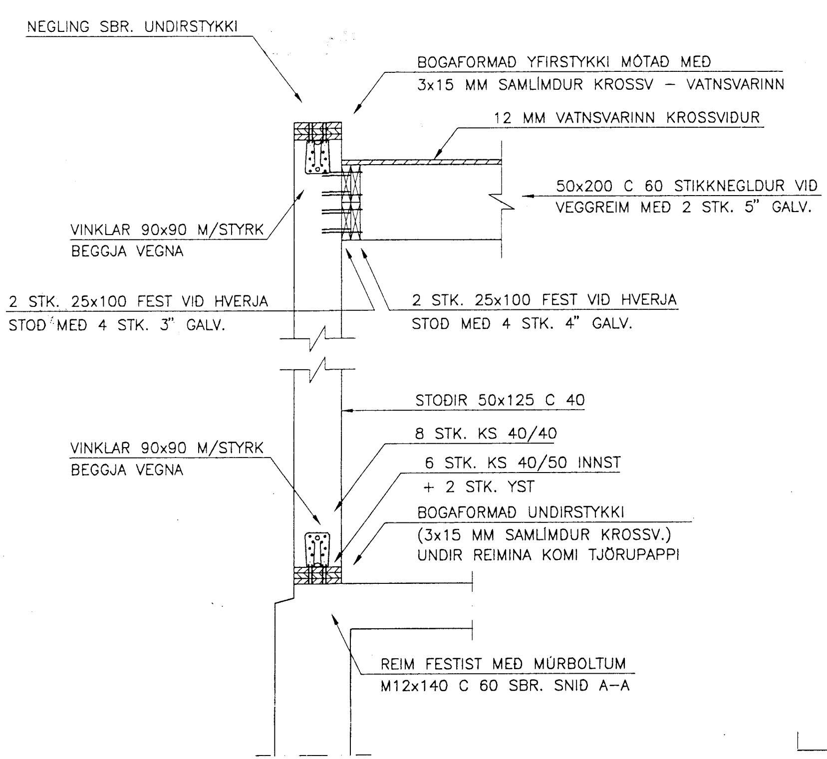
SNID D-D 1:10
