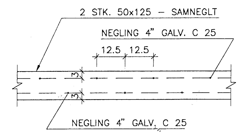
SAMNEGLING TVÖFALDRA STODA 1:10
