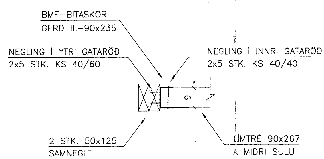
DEILI D6 1:10
