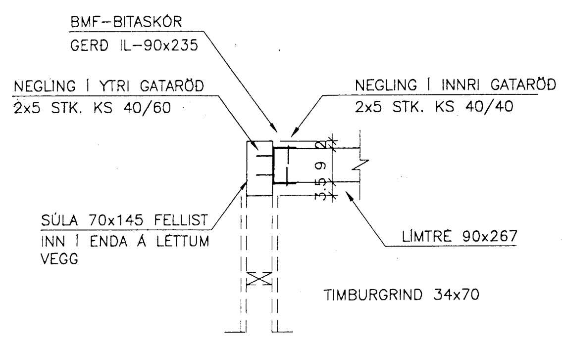
DEILI D5 1:10
