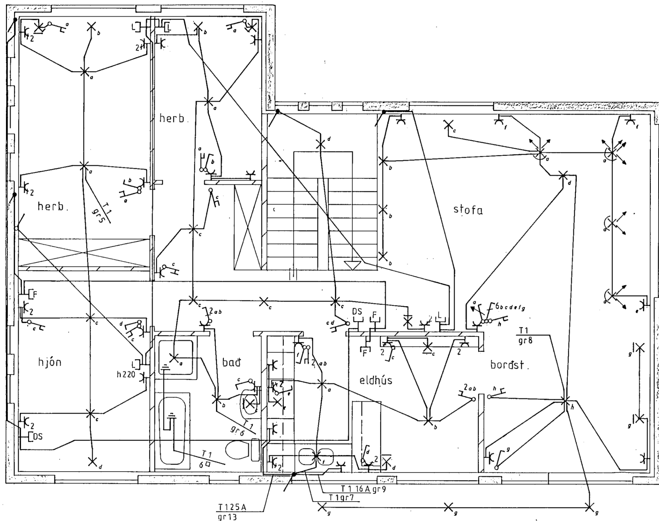
Grunnmynd efri hæðar mkv. 1:50
