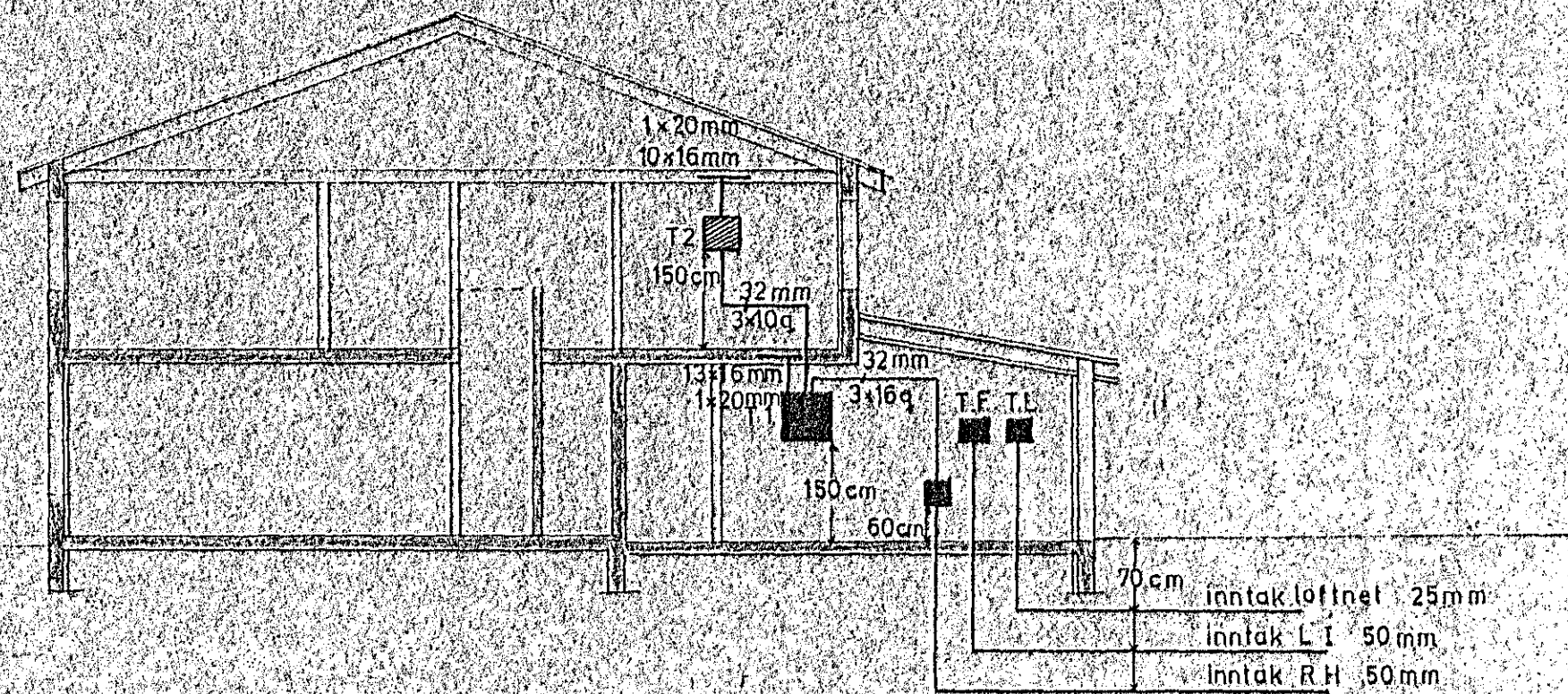
SNID A-A 1:100
