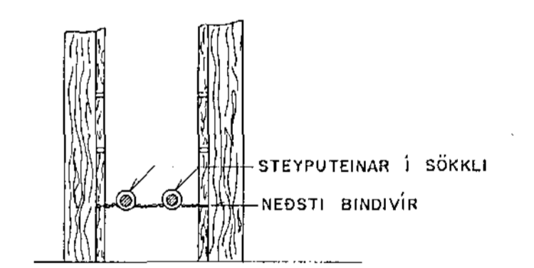
SNID A-A
