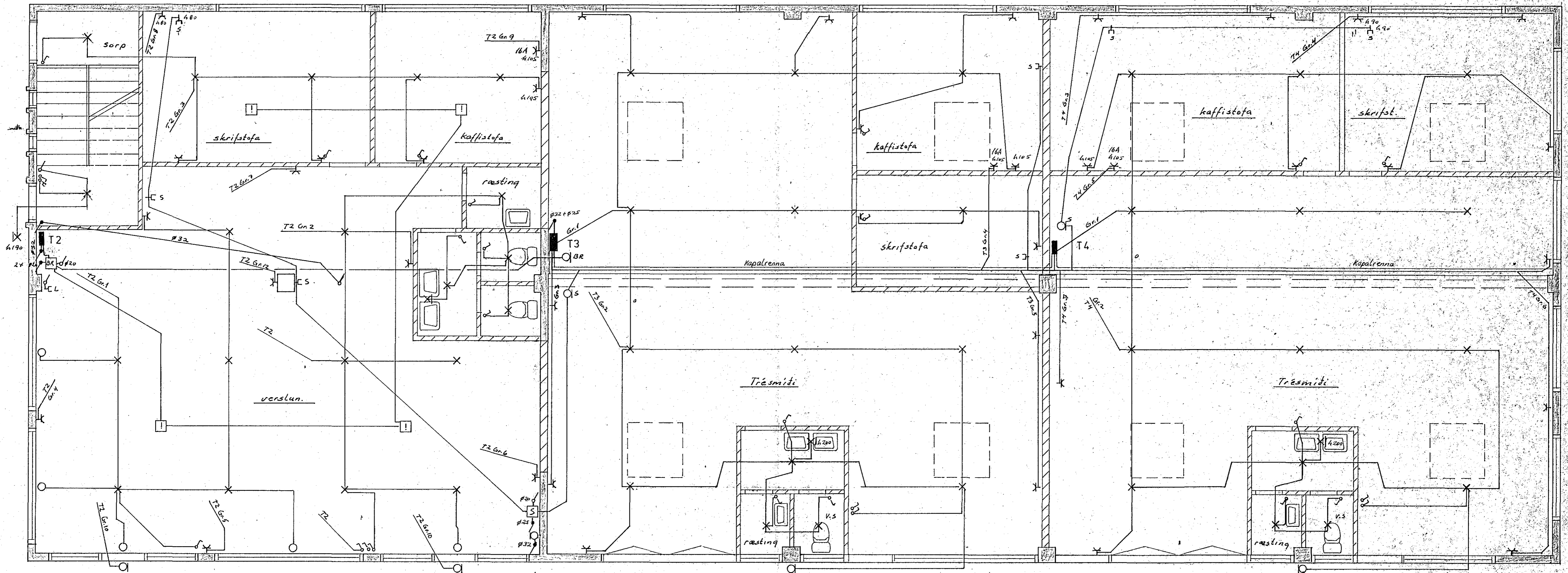
GRUNNMYND 1. HÆÐAR M. 1:50
