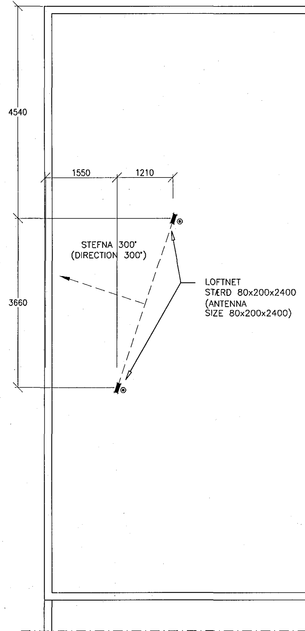
ÞAKMYND LOFTNET MKV 1:50 (ROOF PLAN ANTENNAS SCALE 1:50)
