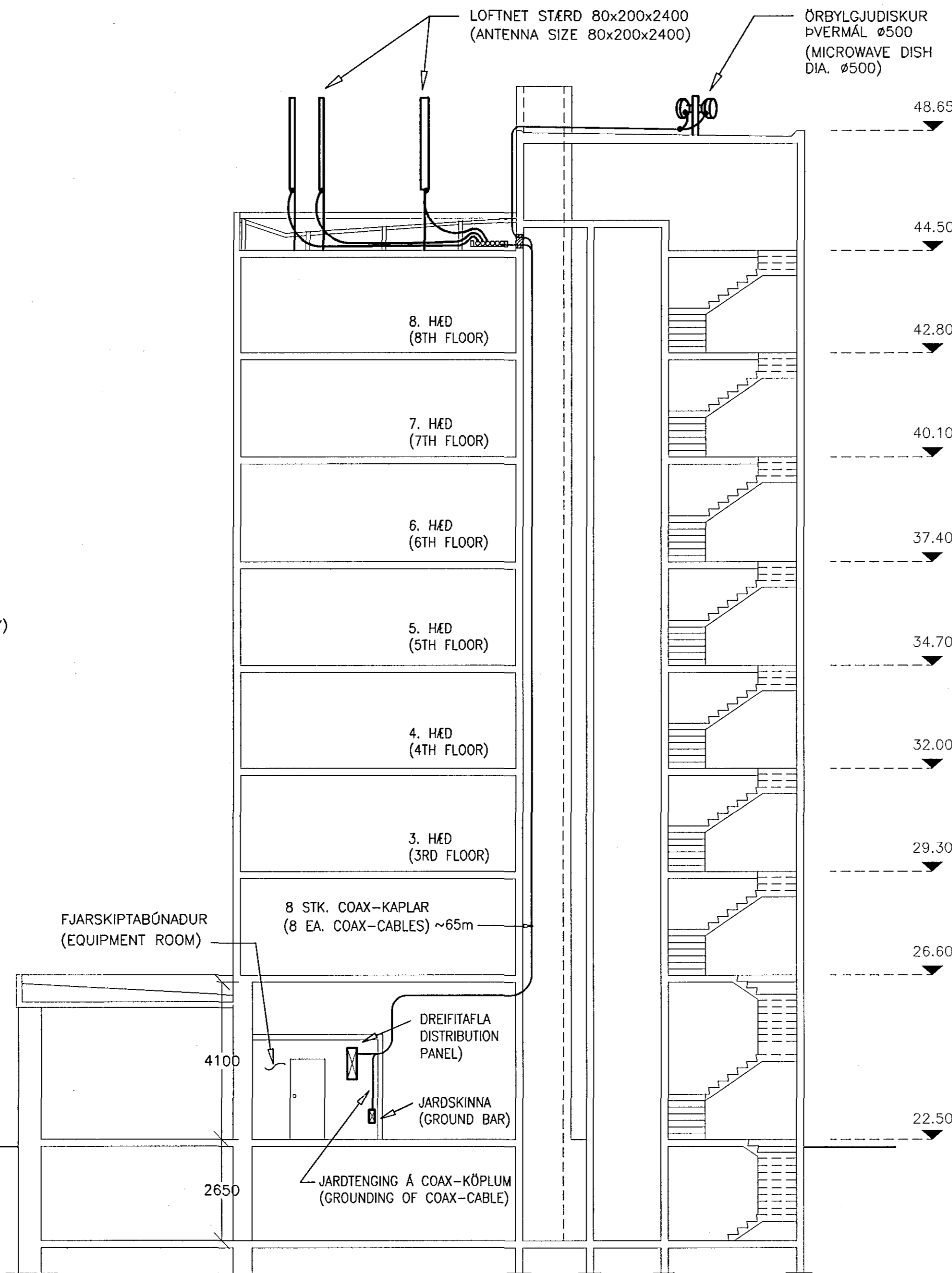
SNIÐ MKV 1:100 (SECTION SCALE 1:100)
