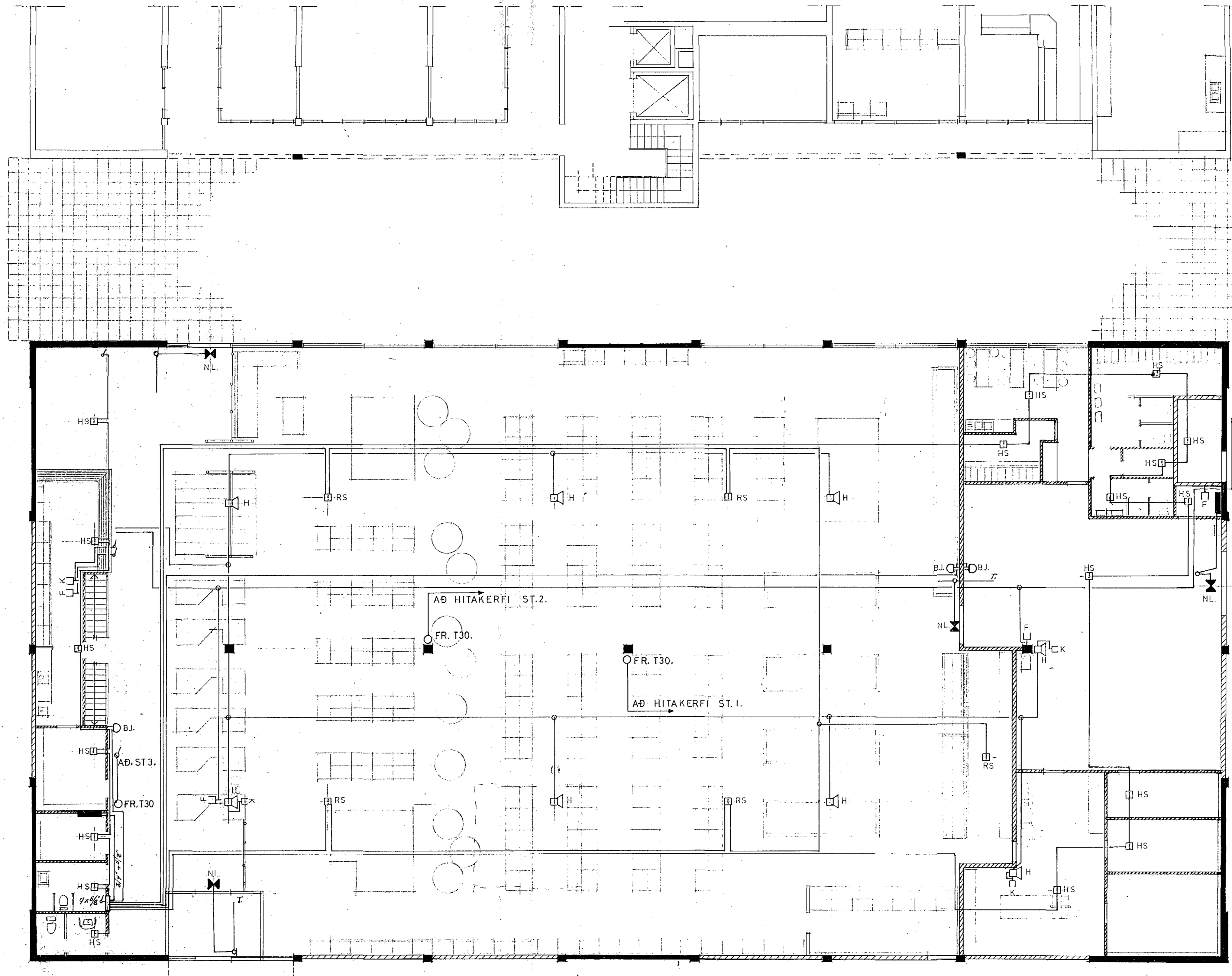
1. HÆÐ HULIÐ LÖGN
