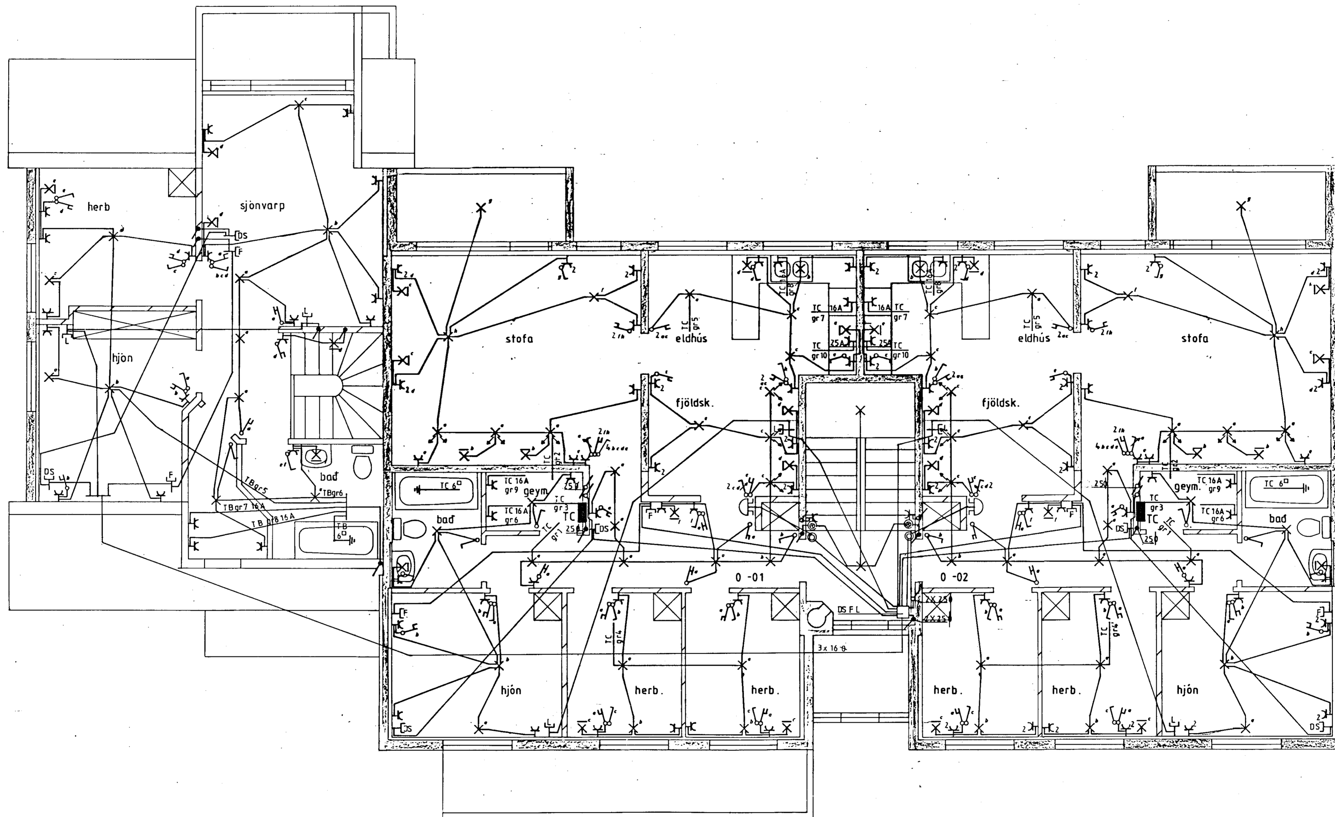
Grunnmynd 2 hæð mkv.1:50
