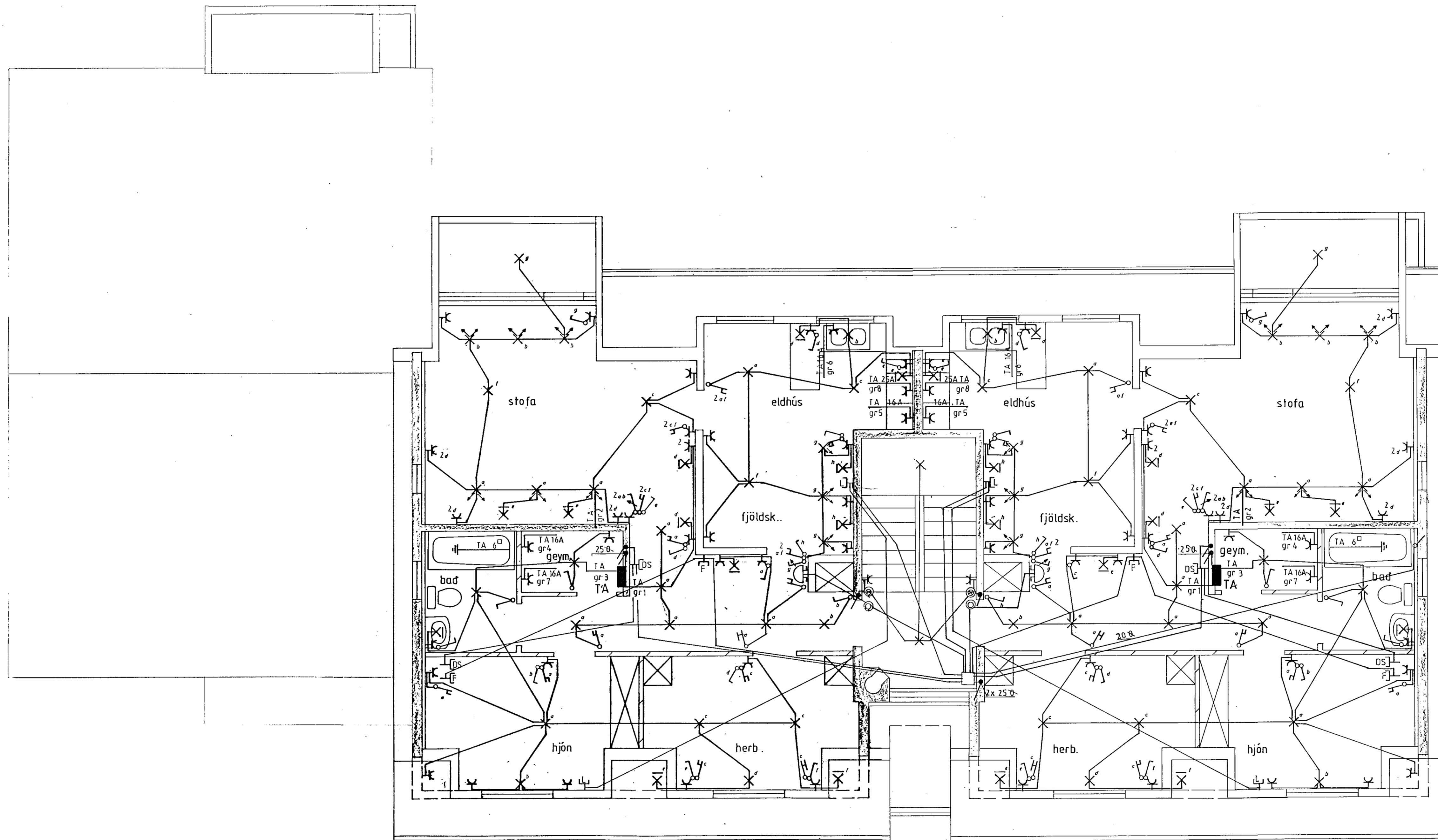
Grunnmynd ris mkv 1:50
