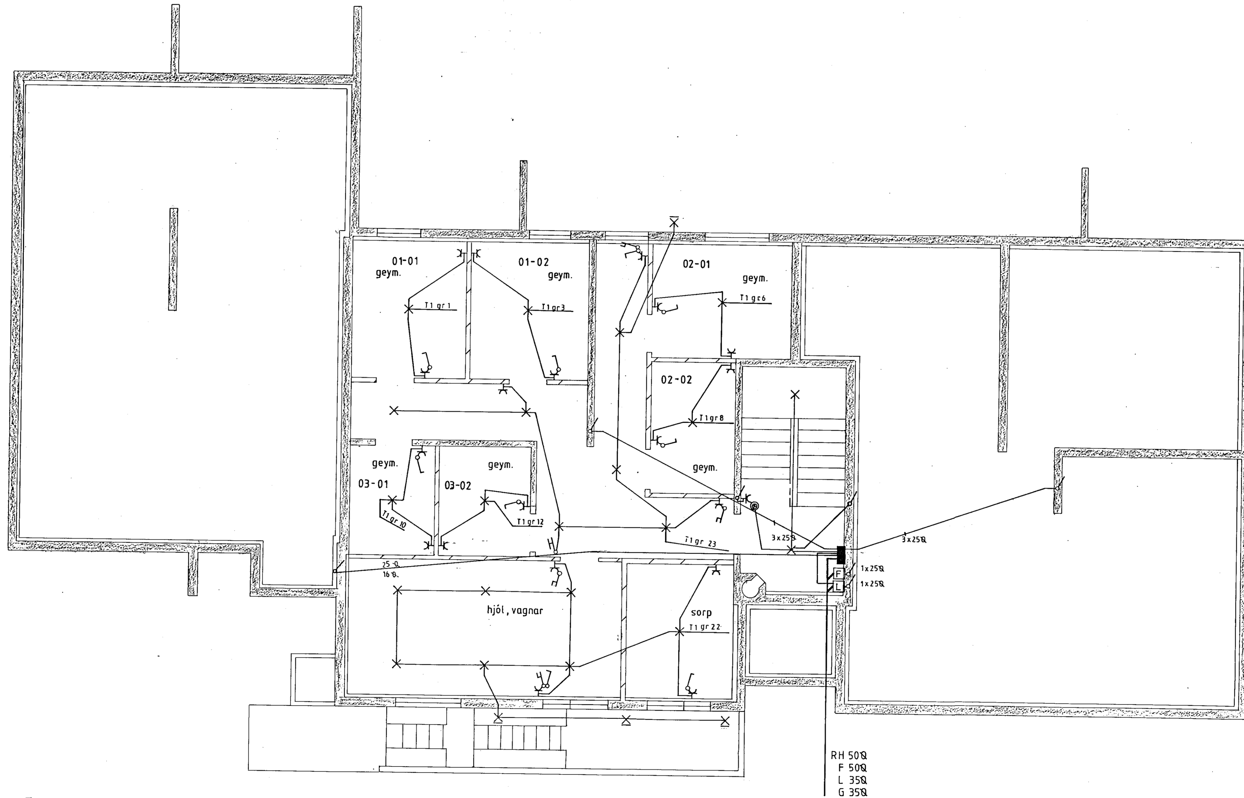
Grunnmynd kjallara mkv.1:50
