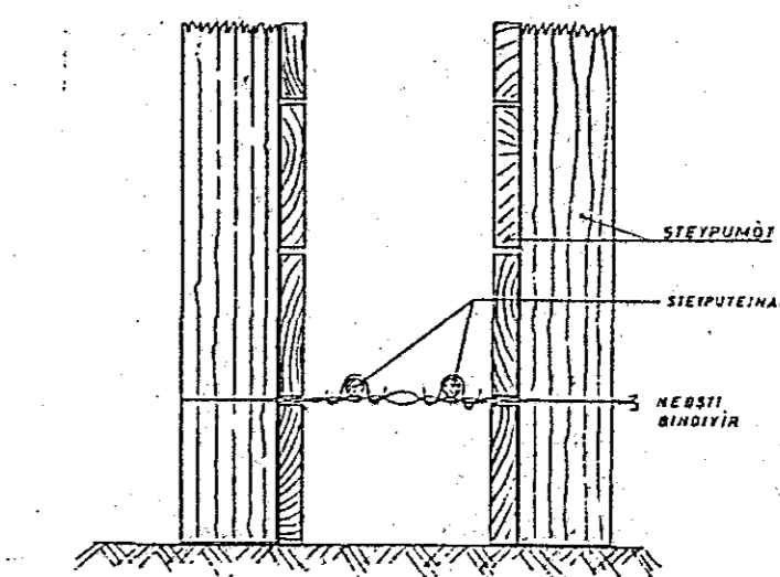
SNID A-A Í SÖKKULVEGG
