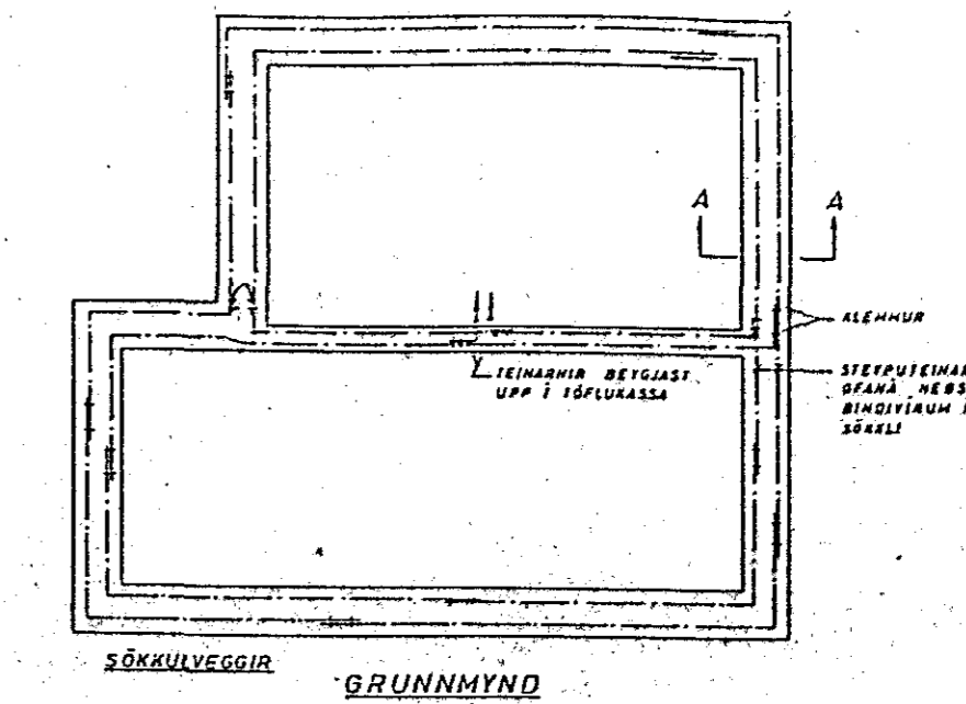
SÖKKULVEGGIR GRUNNMYND
