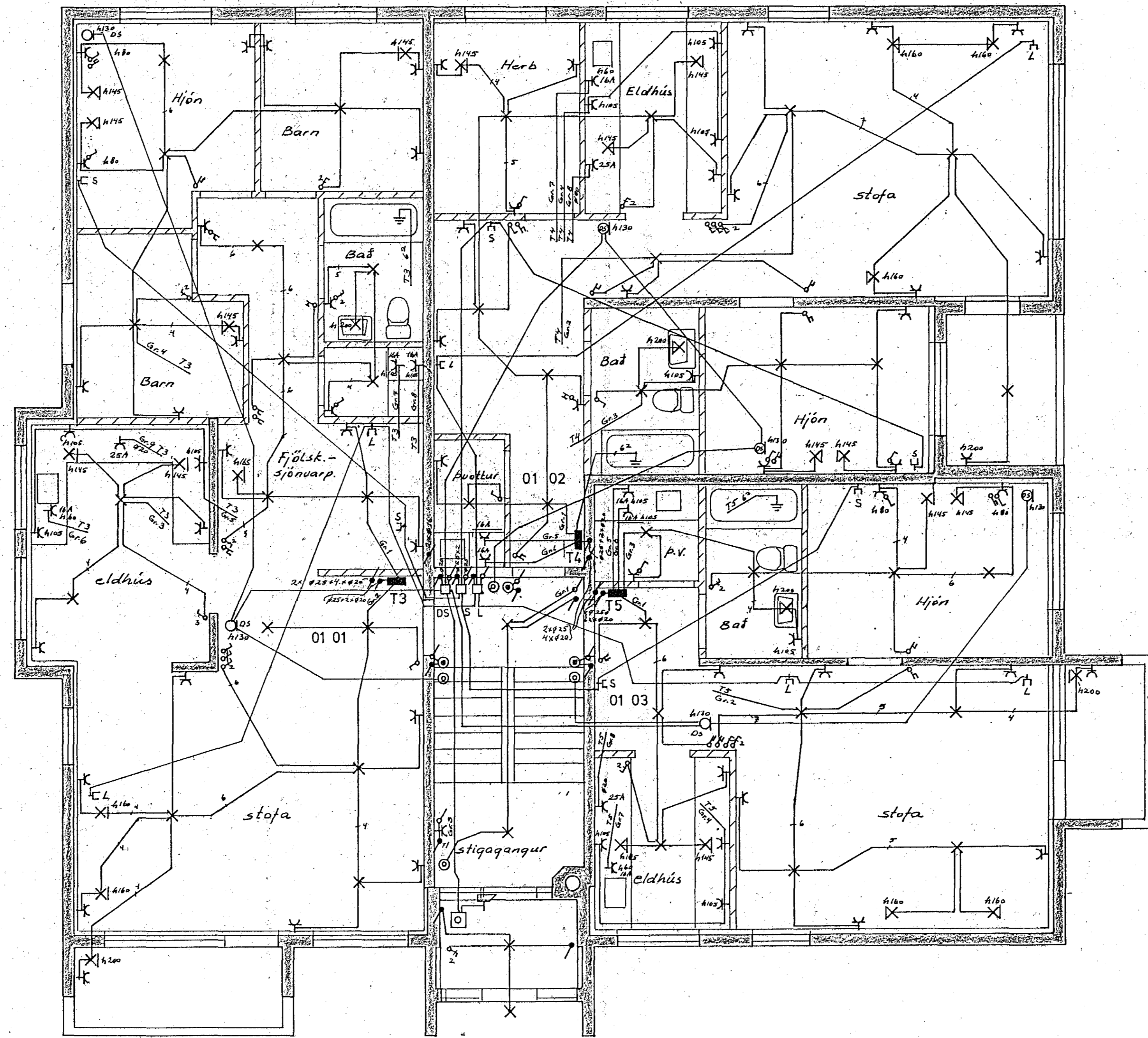
GRUNNMYND 1. HÆÐAR M. 1:50
