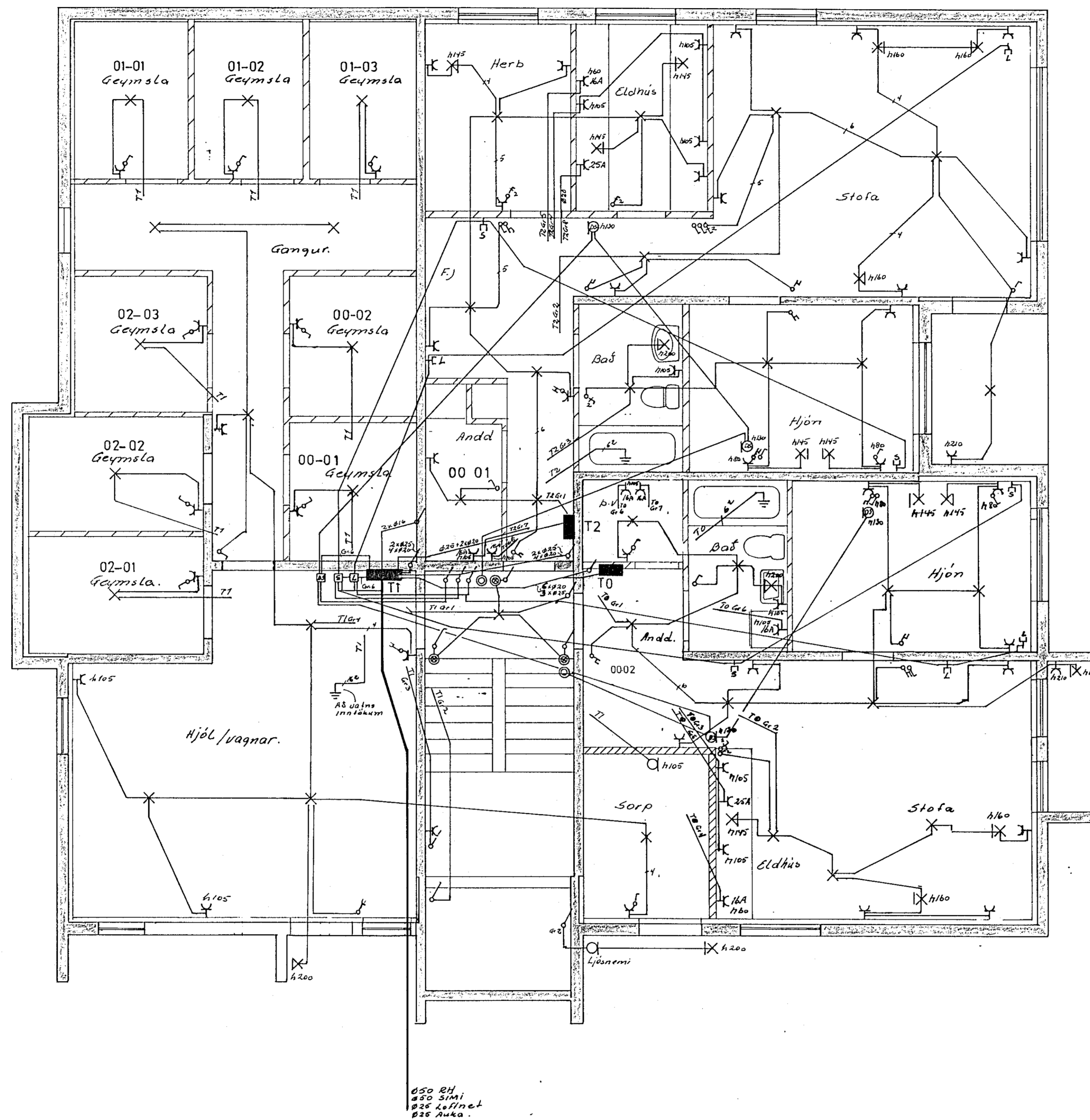
GRUNNMYND JARÐHÆÐ M. 1:50
