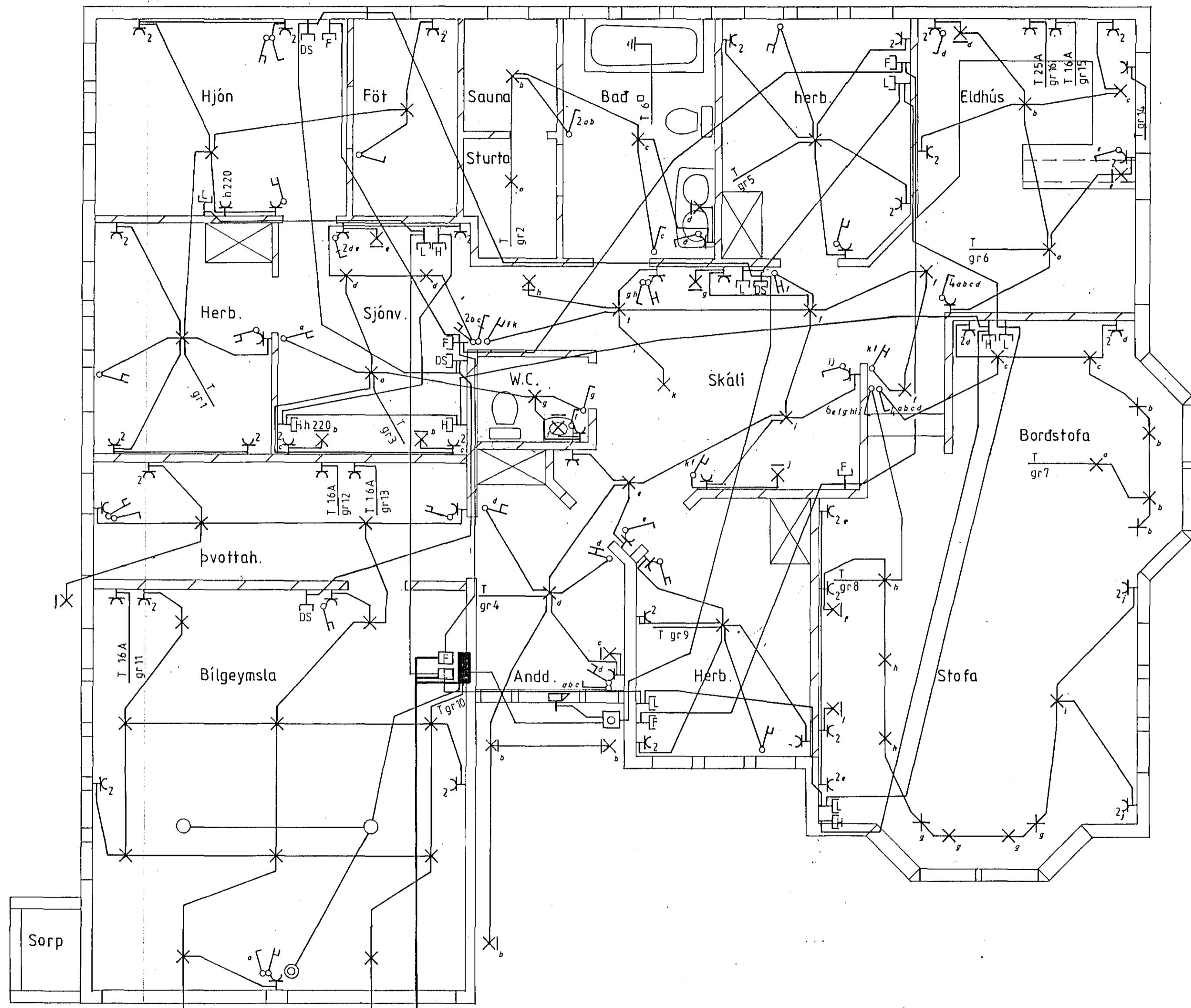
Grunnmynd mkv. 1:50
