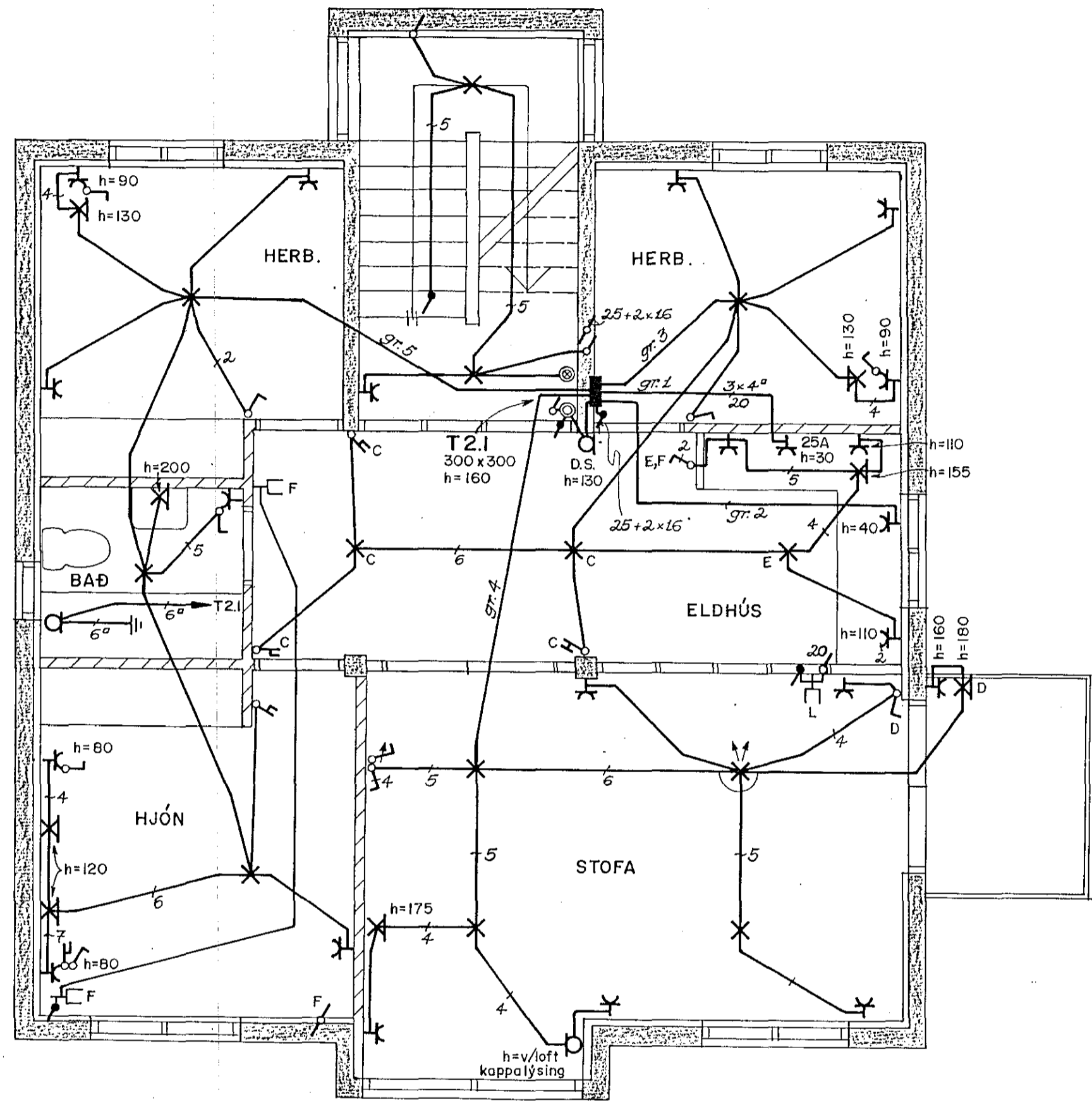
2. HÆÐ
