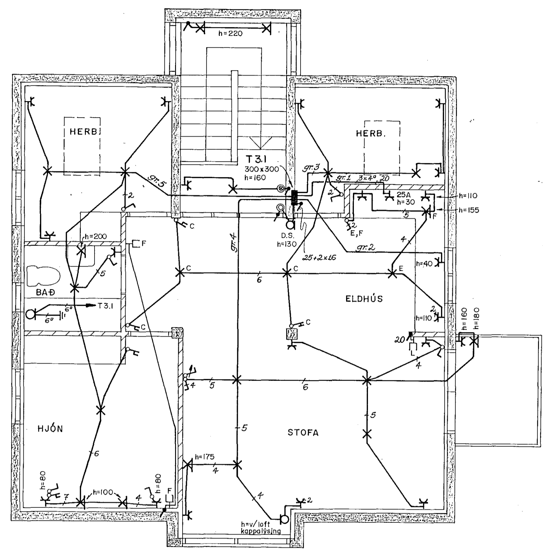
3. HÆÐ
