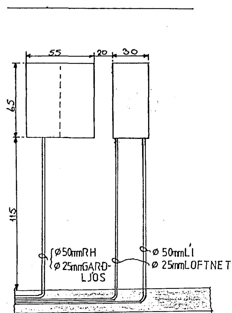
SNID A-A
