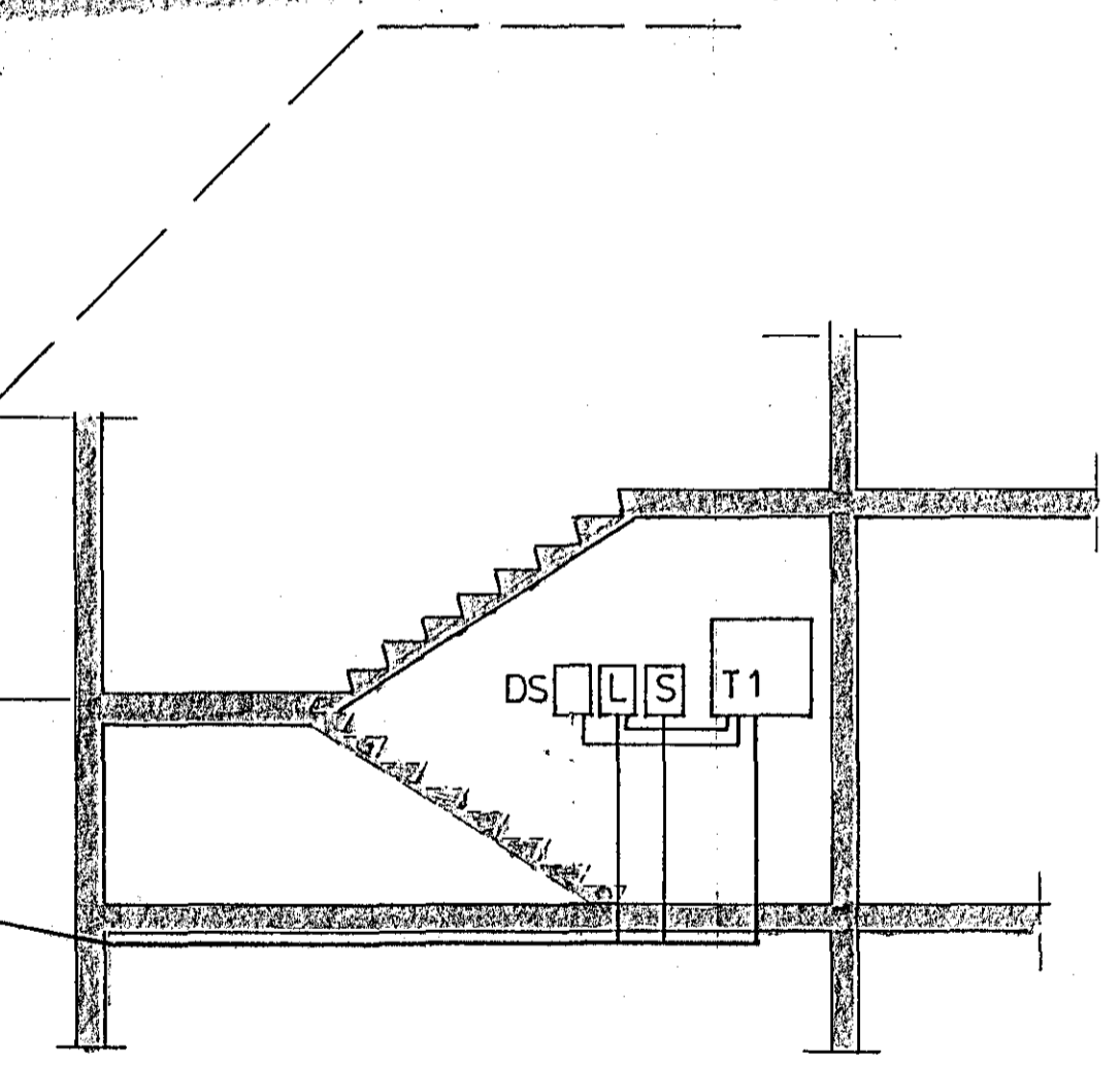
Sneiðing M 1:50
