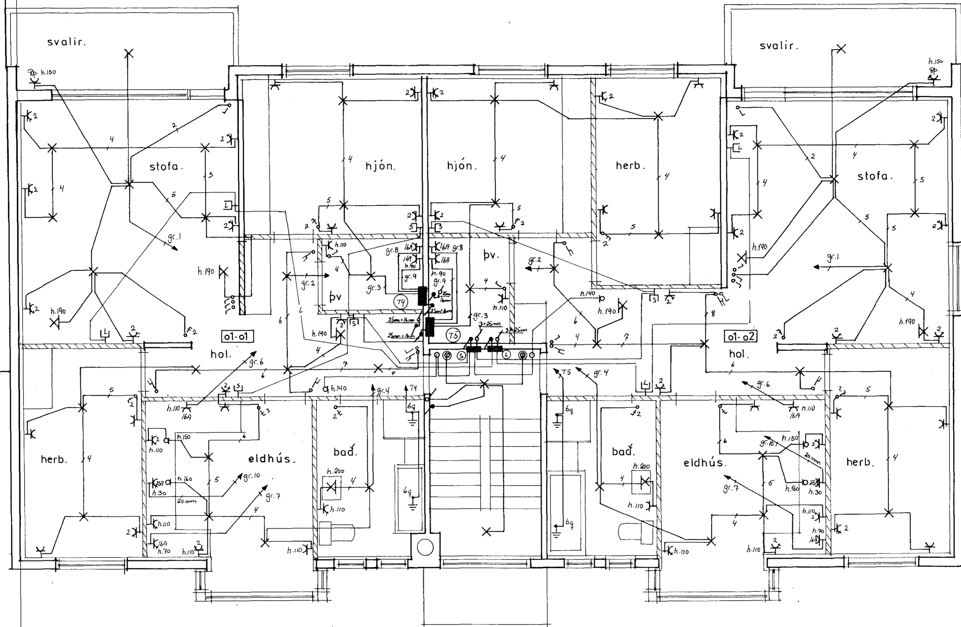
GRUNNMYND 1. HÆÐ MÁL 1:50
