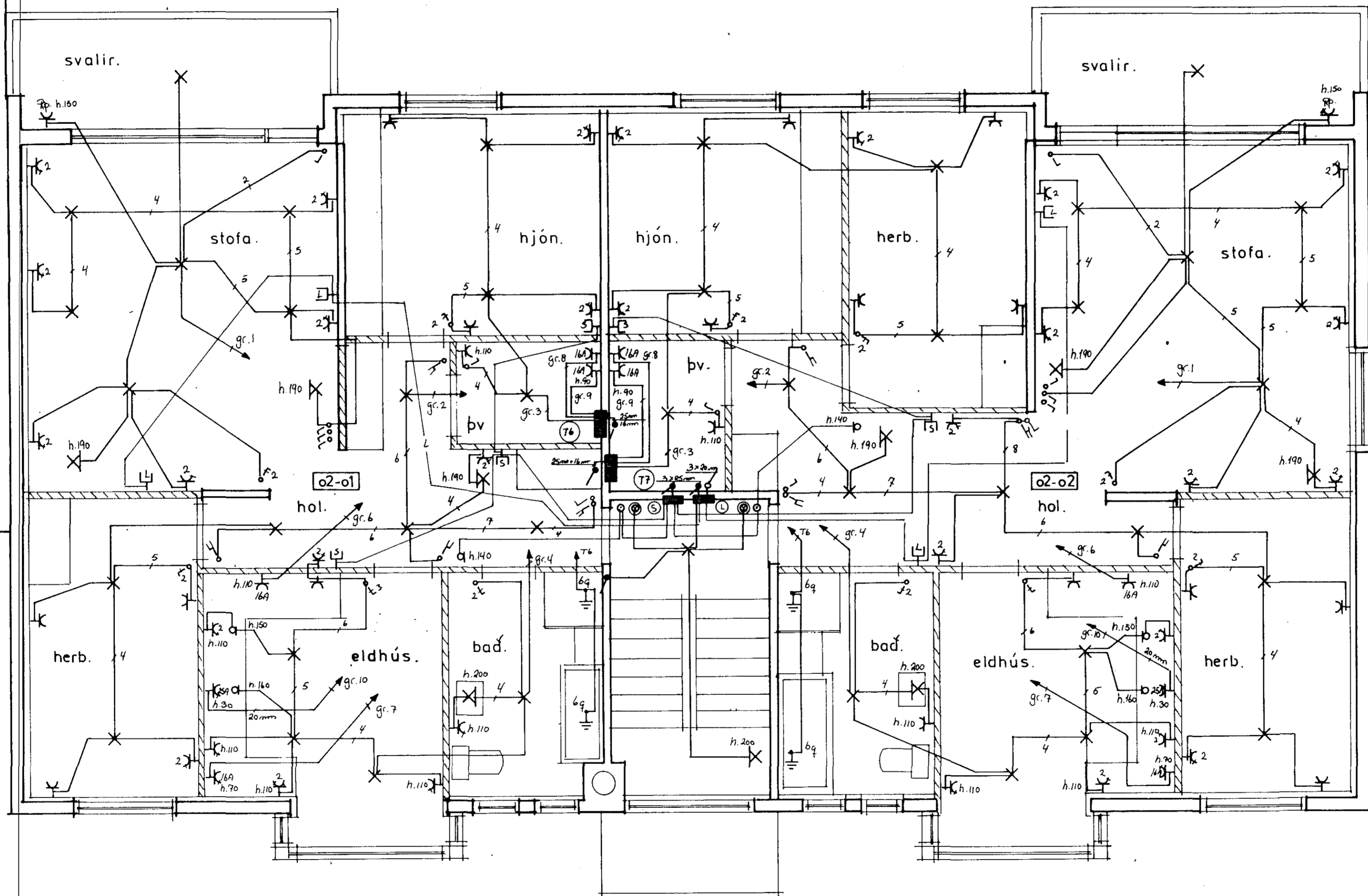
GRUNNMYND 2. HÆÐ MÁL 1:50
