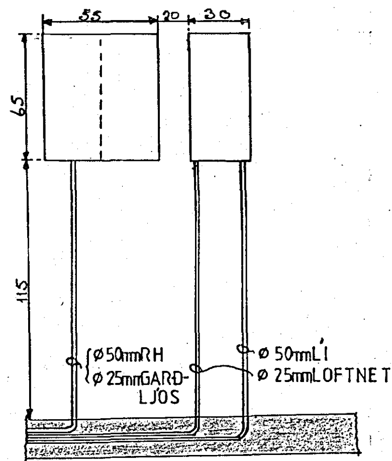
SNID A-A
