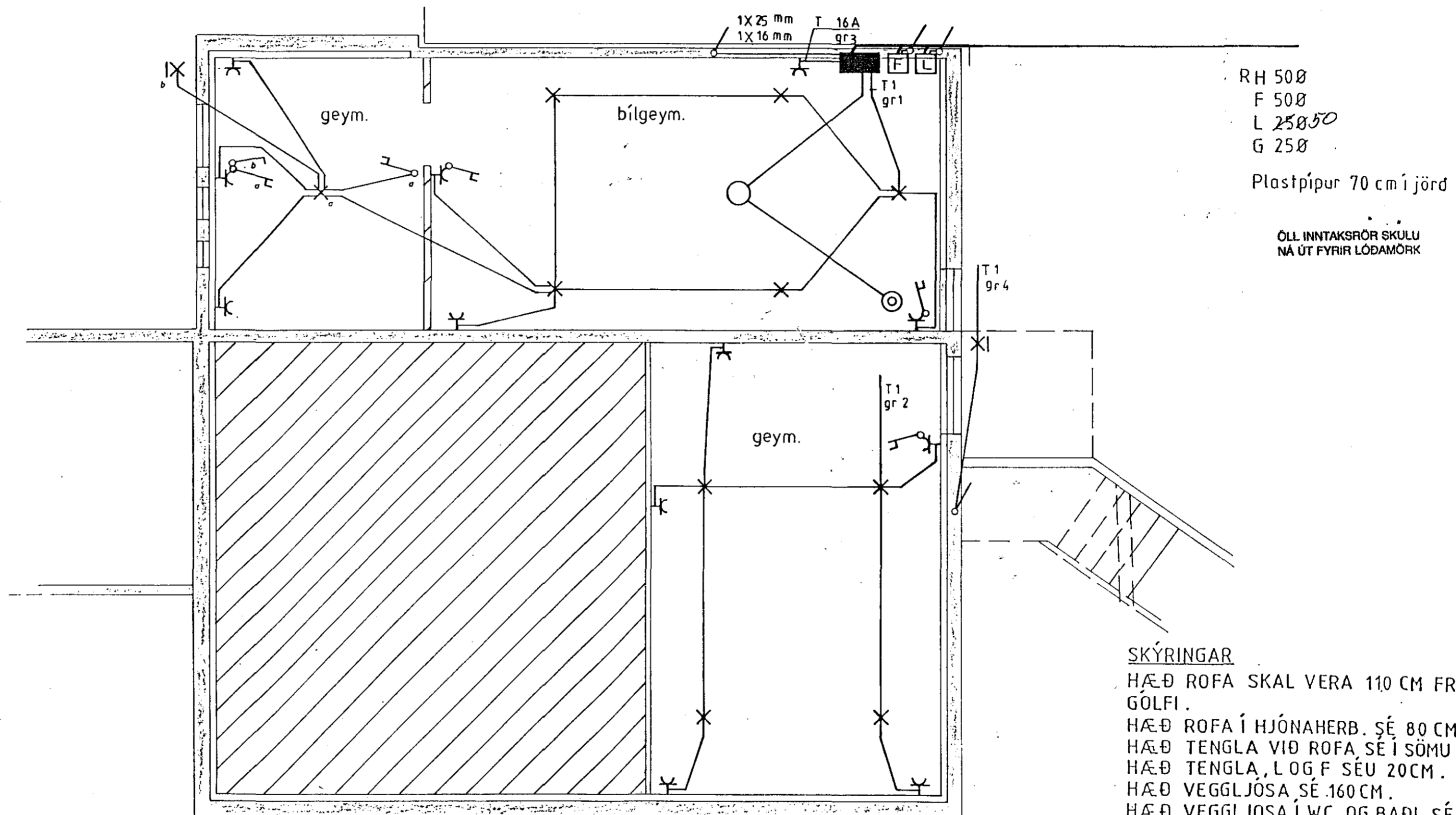
Grunnmynd kjallara mkv 1:50
