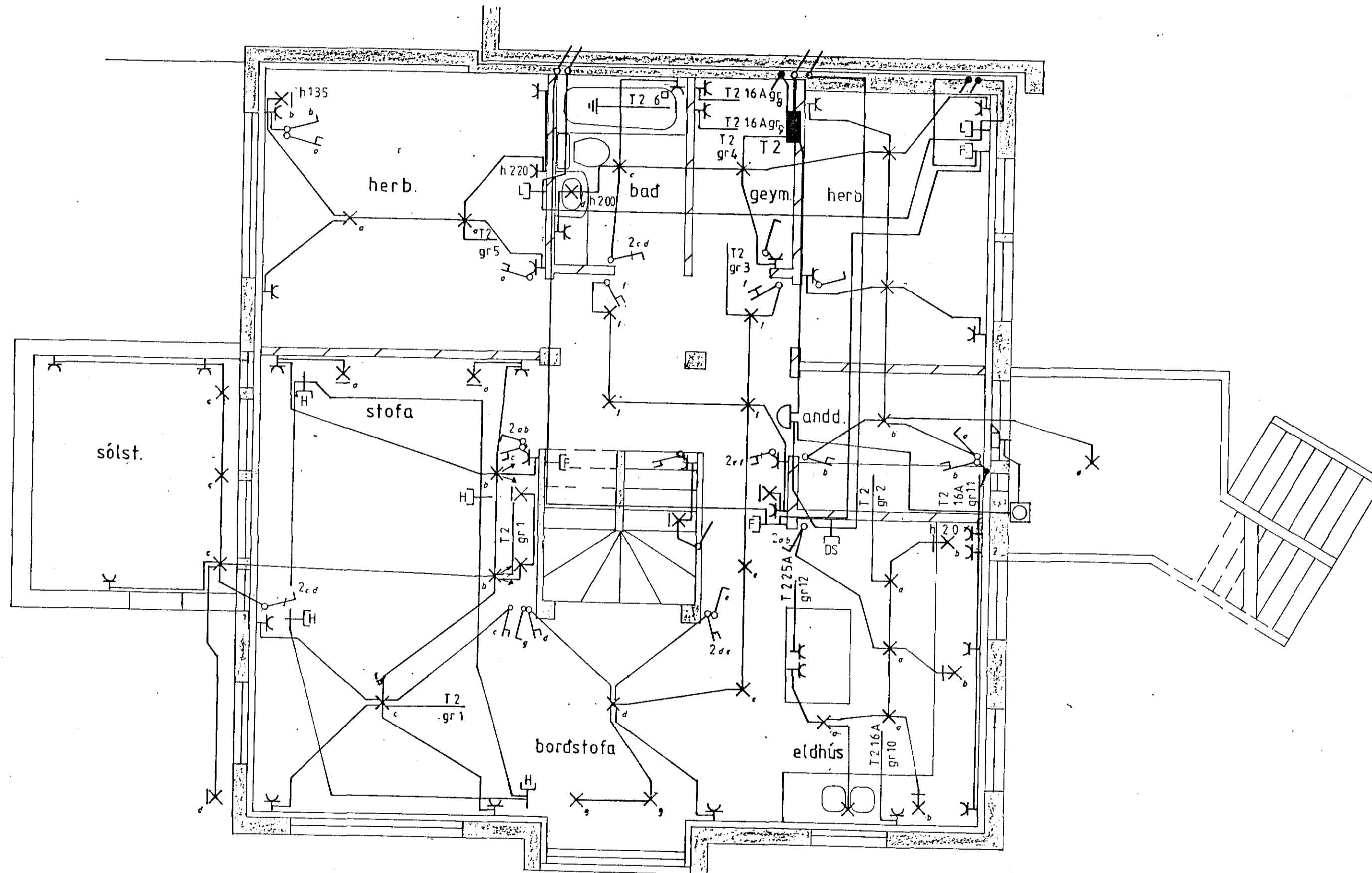
Grunnmynd hæðar mkv. 1:50
