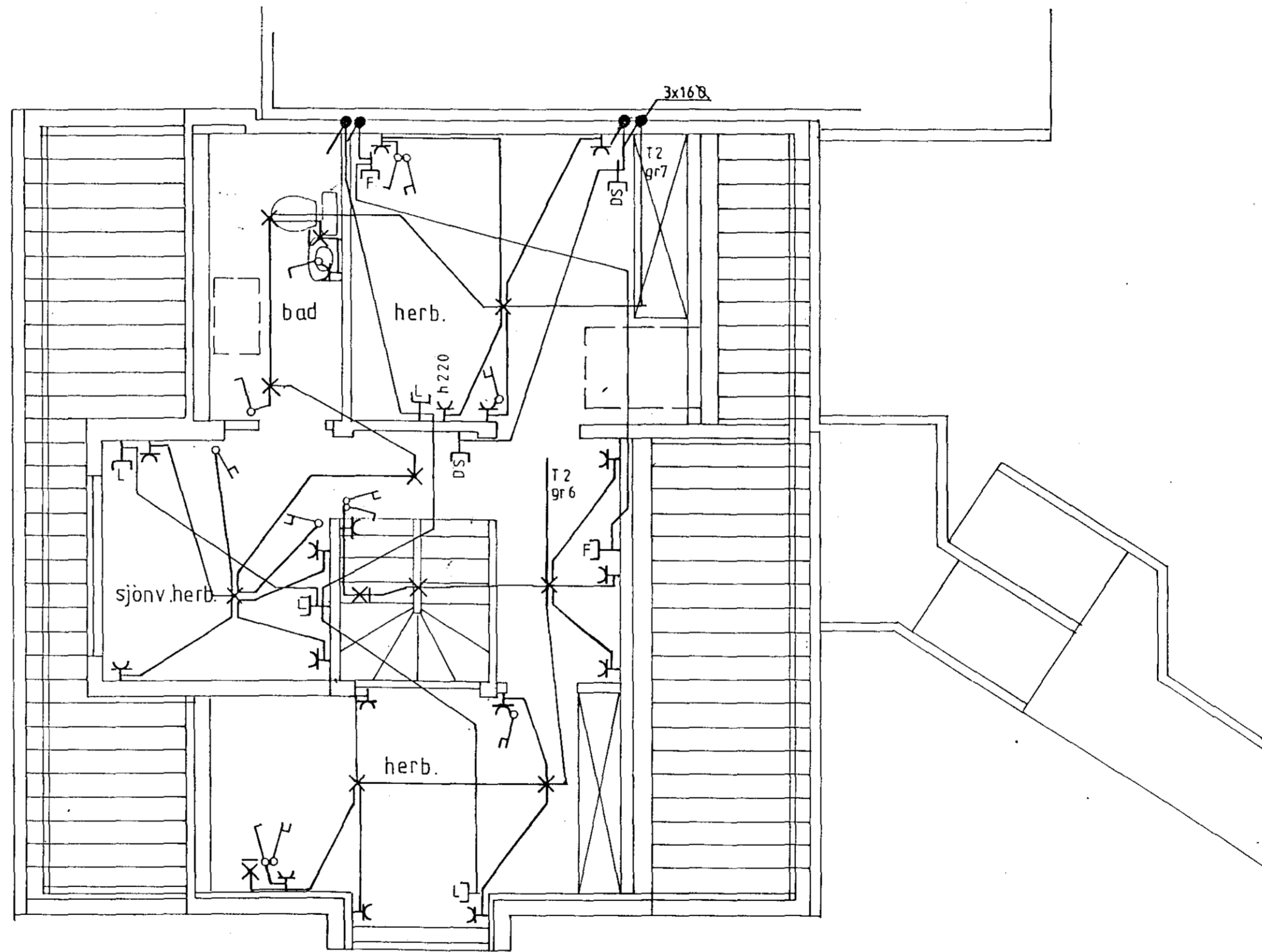
Grunnmynd ris mkv. 1:50
