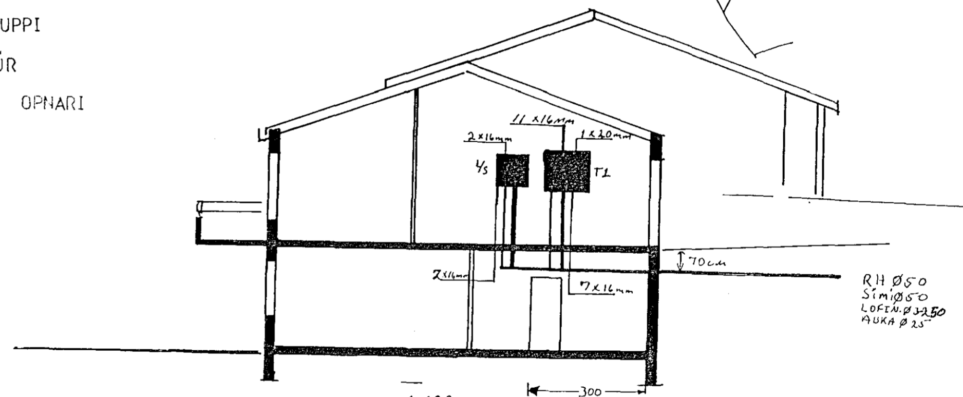
1:100 SNÍÐ A-A H-T1 140 H-LÁSPENNUBOX 150
