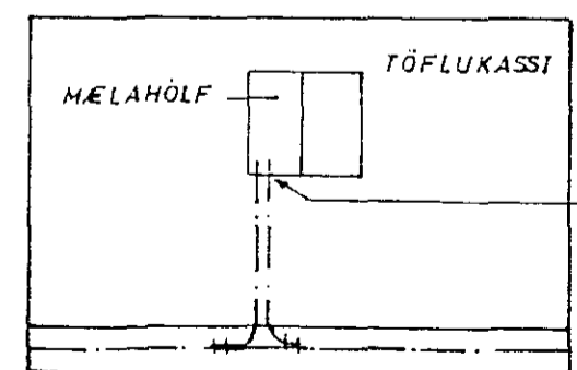
SNID A-A Í SÖKKULVEGG
