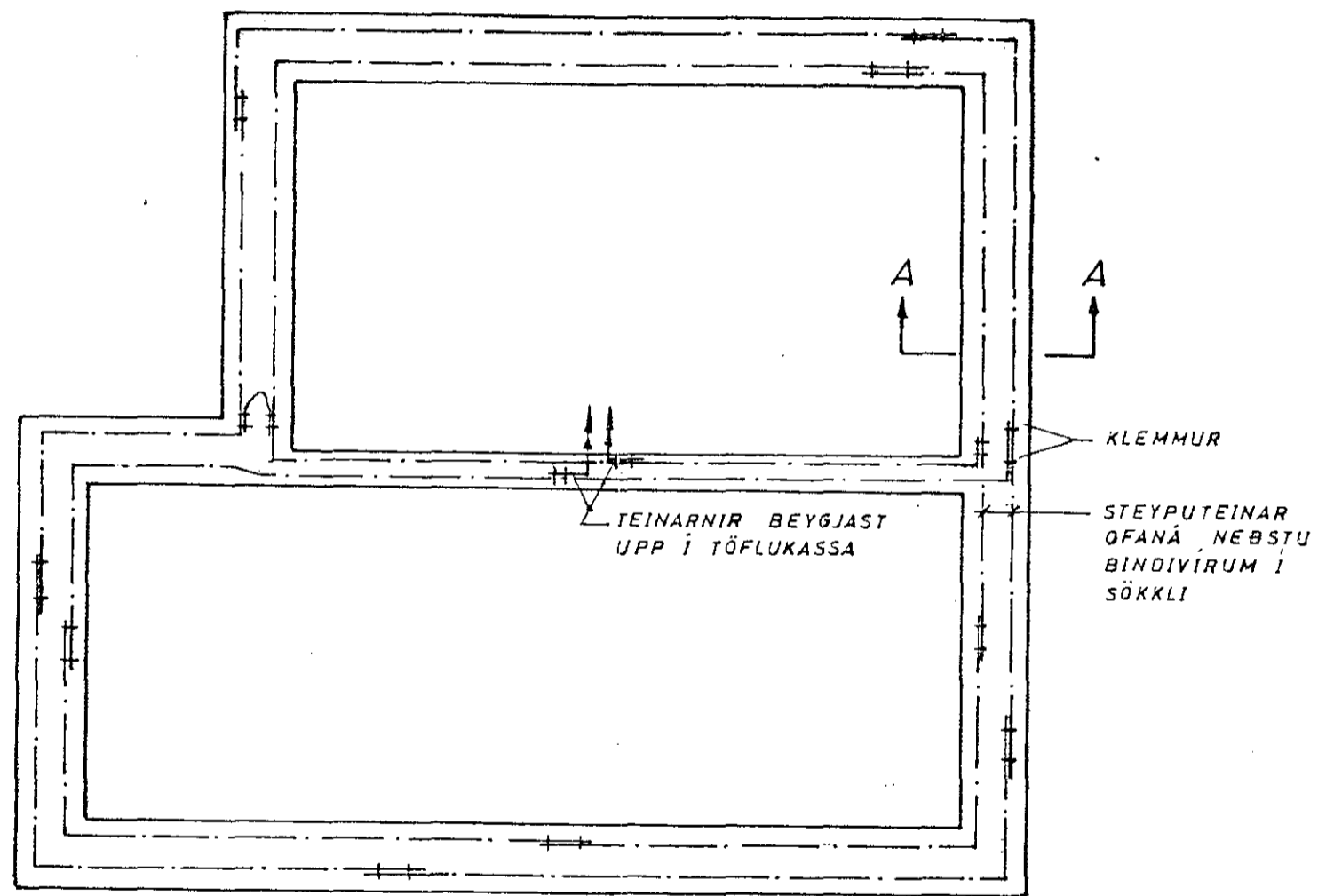
SÖKKULVEGGIR GRUNNMYND
