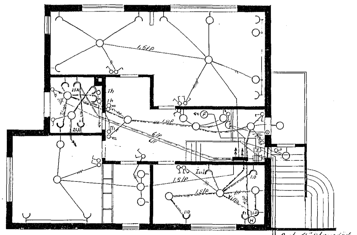
I. Hæð 2. sl. 4" stennir fyrir rafmagn síma og eldh. gólf
