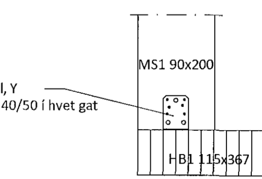
Snið A-A
