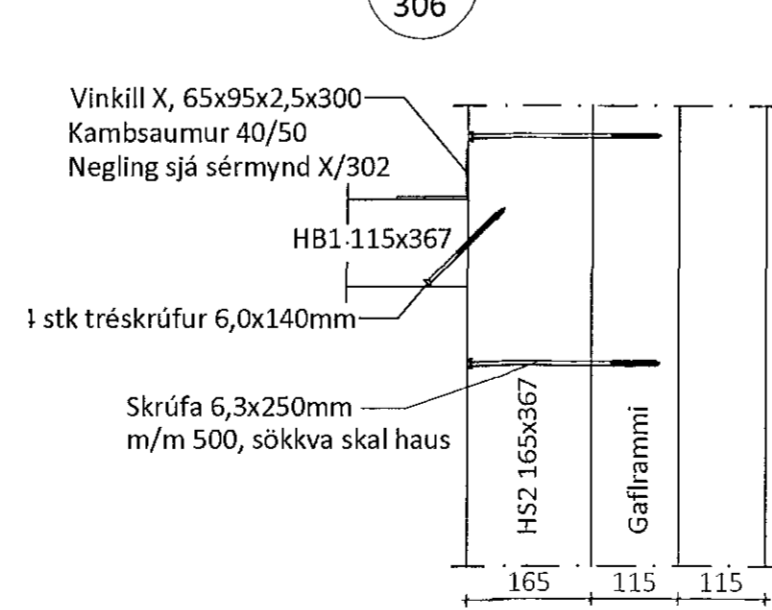
Sérmynd 26 Mkv. 1:10
