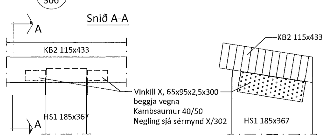
Sérmynd 23 Mkv. 1:10
