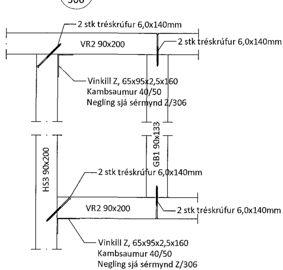
Sérmynd 25 Mkv. 1:10
