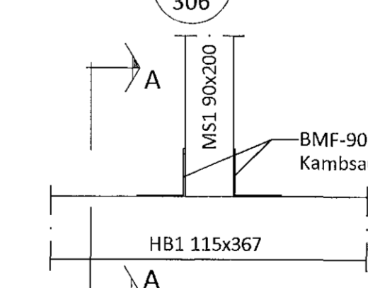
Sérmynd 24 Mkv. 1:10
