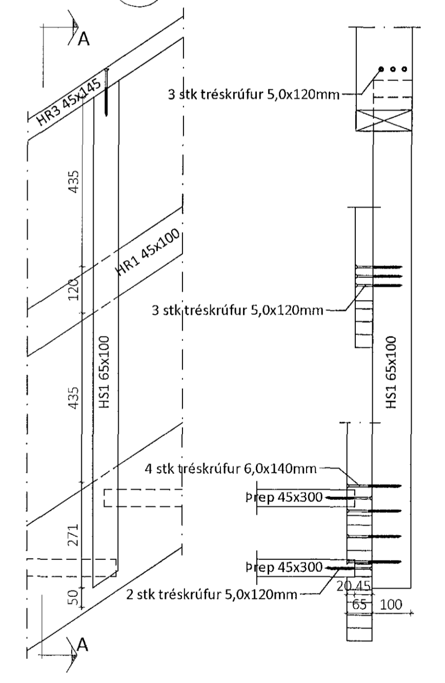
Sérmynd 39 Mkv. 1:10 Sníð A-A 309
