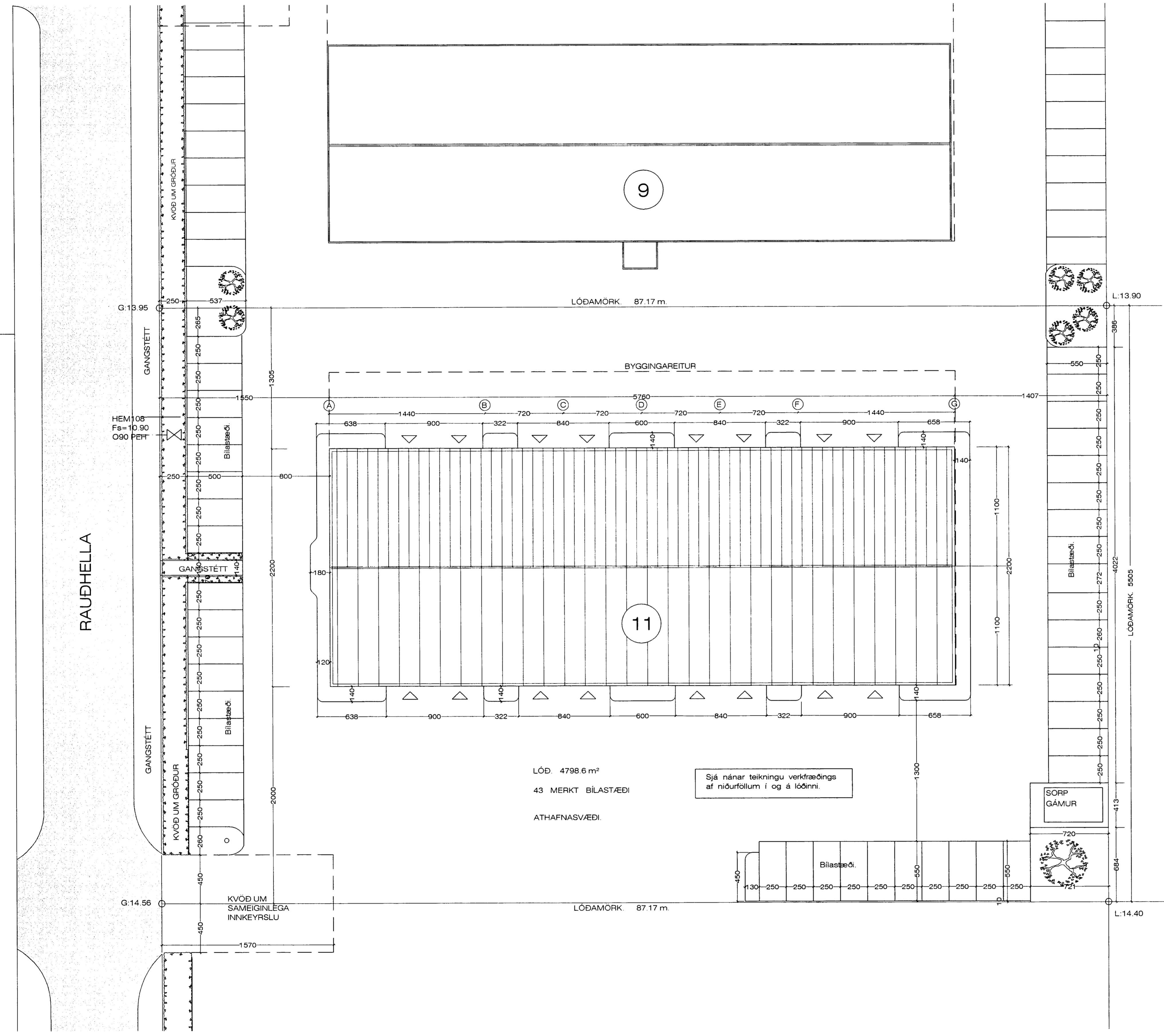
Lóðarteikning. 1:200
