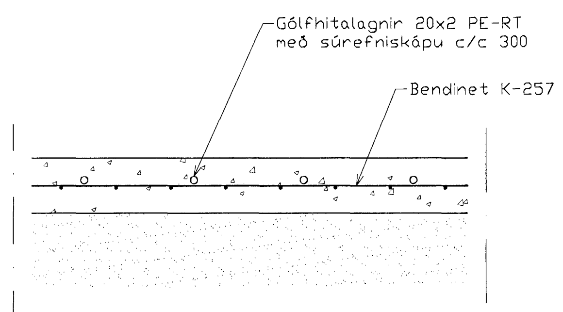
Gólfhiti, Snið 1:10
