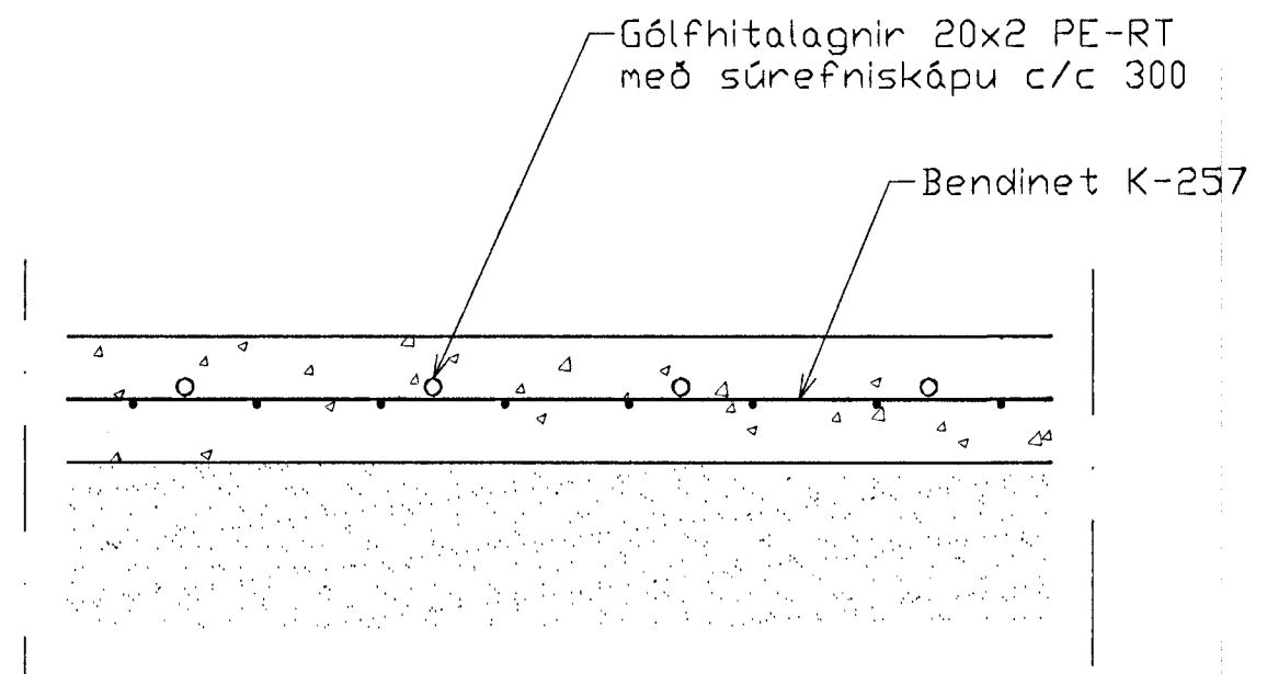
Gólfhiti, Snið 1:10
