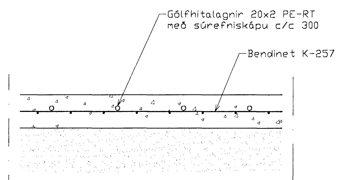
Gólfhiti, Snið 1:10
