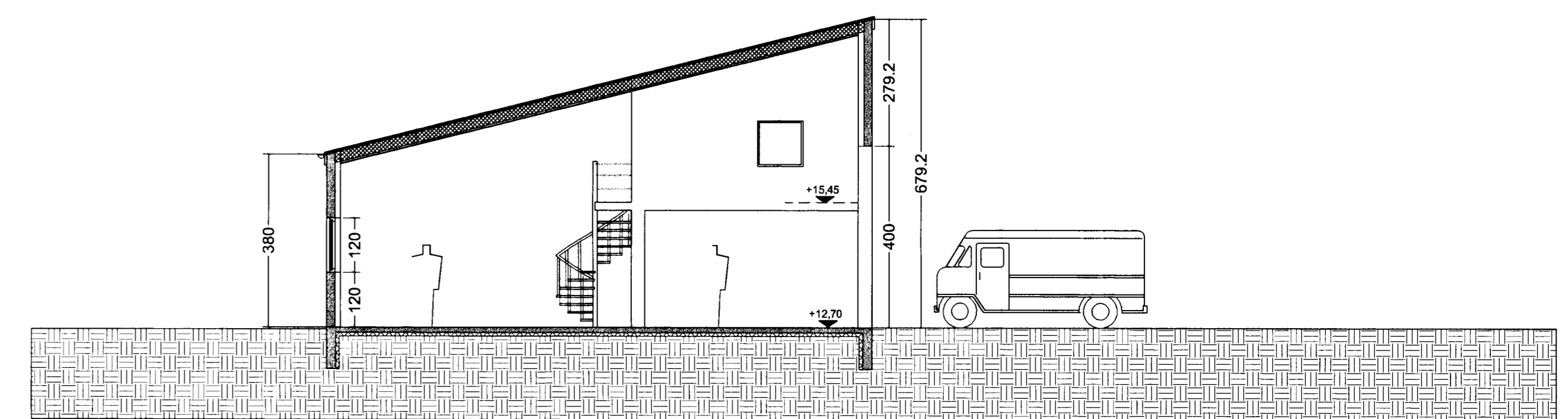
SKURÐUR B-B
