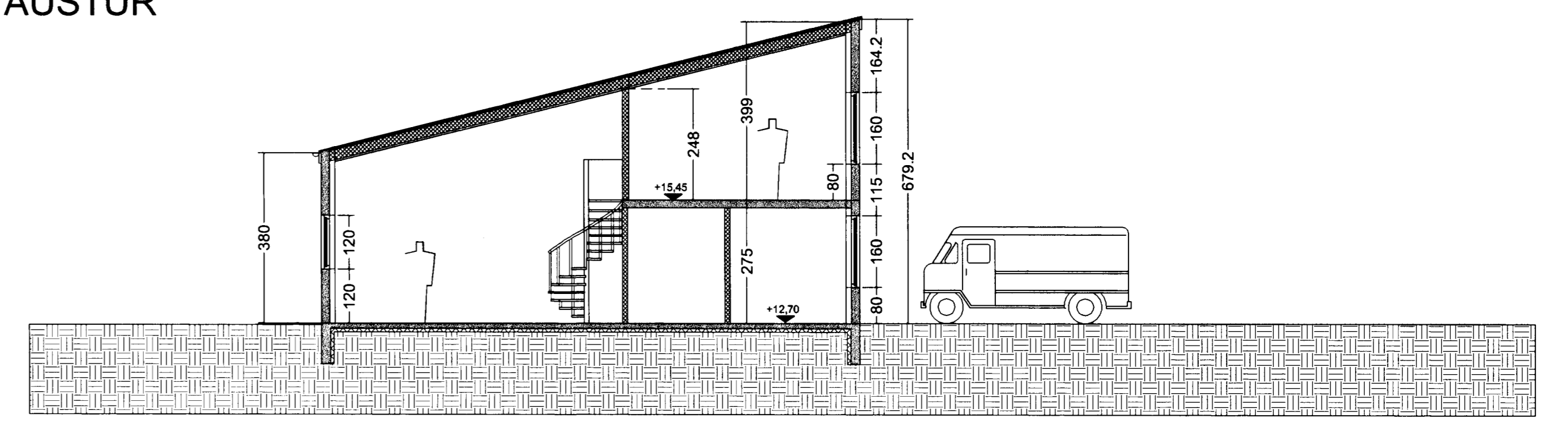
SKURÐUR A-A
