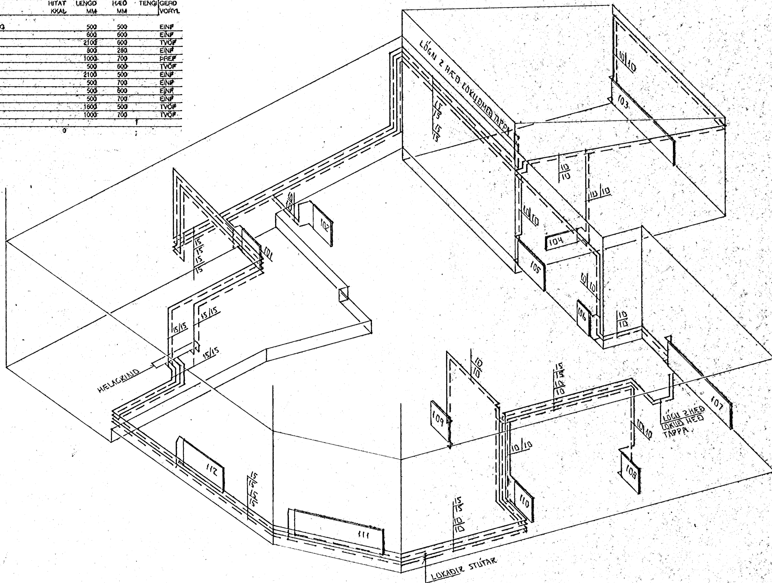
RÚMMYND - HITALAGNA 1 : 50
