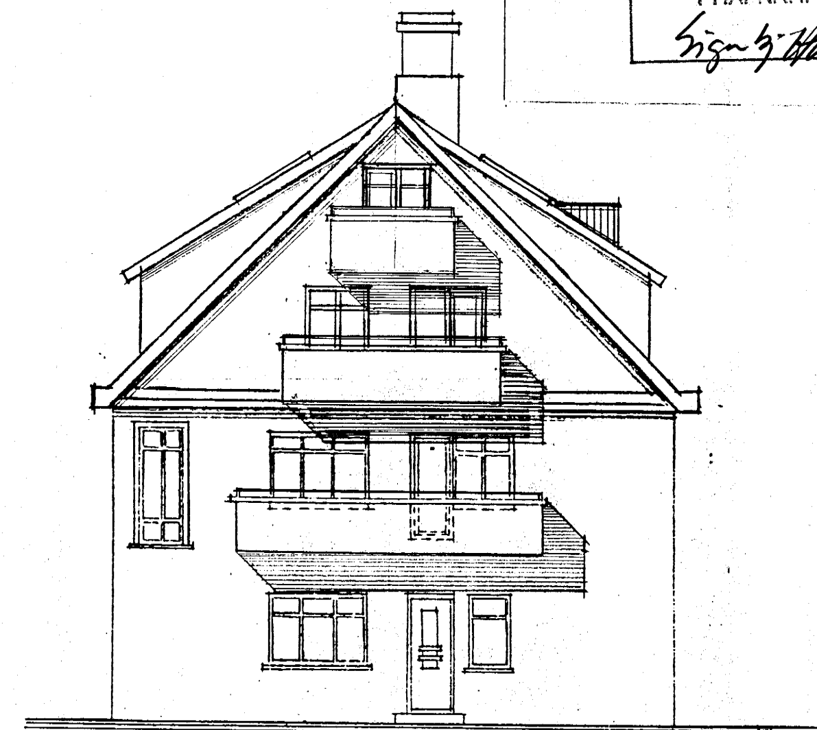
SUDVESTUR 1:100
