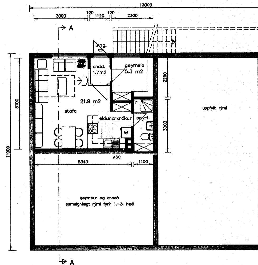
Grunnmynd kjallara mkv. 1:100
